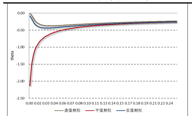
图表 15: Theta 与剩余期限的关系
