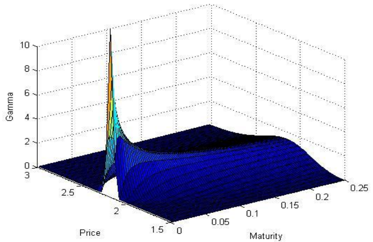
图表 10: Gamma 与标的资产价格、剩余期限的三维图
