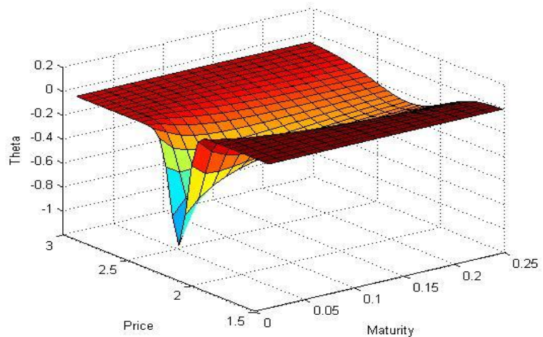
图表 13: Theta 与标的资产价格、剩余期限的三维图
