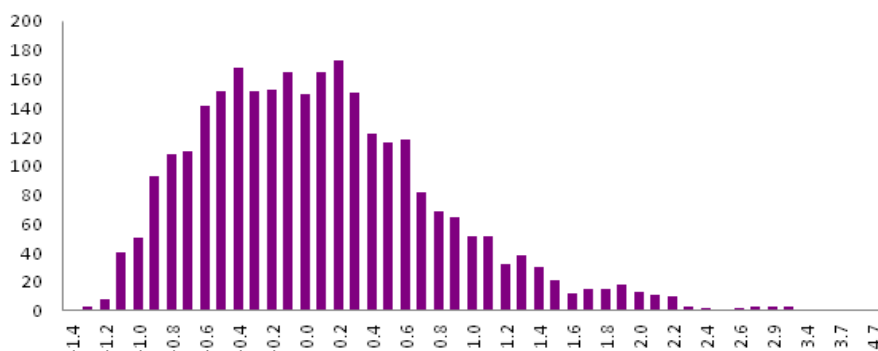
图 20: RRSR 右偏修正标准分分布
