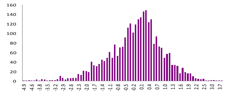
图 14: RSRRS 标准分布
