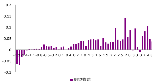
图 22: RRSR 右偏标准分对应其后未来 10 日预期收益
