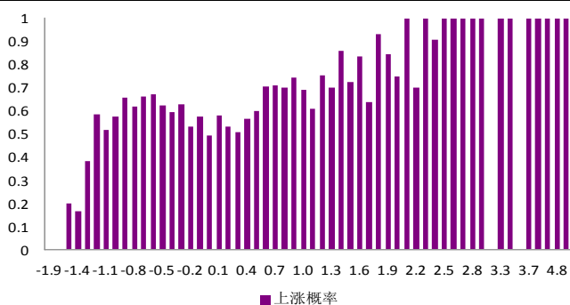
图 21: RRSR 右偏标准分对应其后未来 10 日上涨概率
