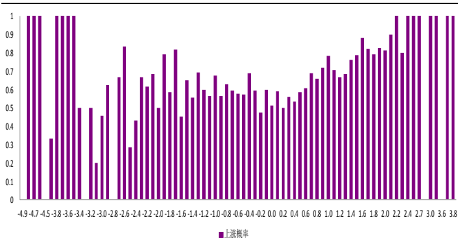
图 16: RSRS 标准分对应其后 10 日上涨概率
