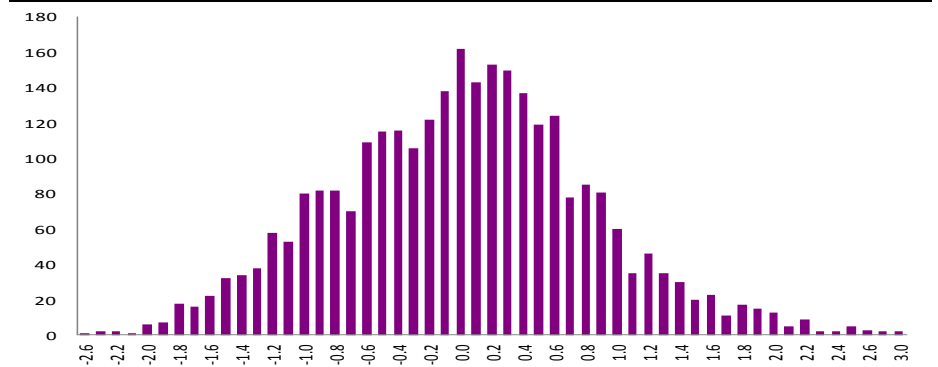
图 15: RSRRS 修正标准分布
