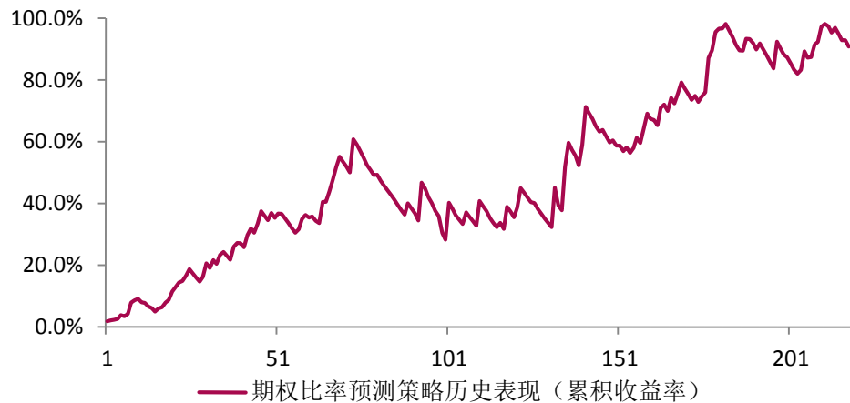
图 8: 期权比率预测策略历史表现 (自 2015 年 2 月 9 日起)
