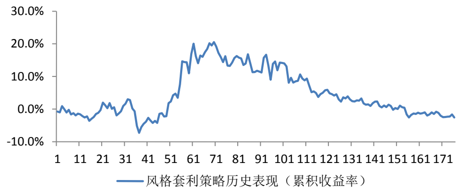
图1: 风格套利策略历史表现 (自2015年4月16日起)
