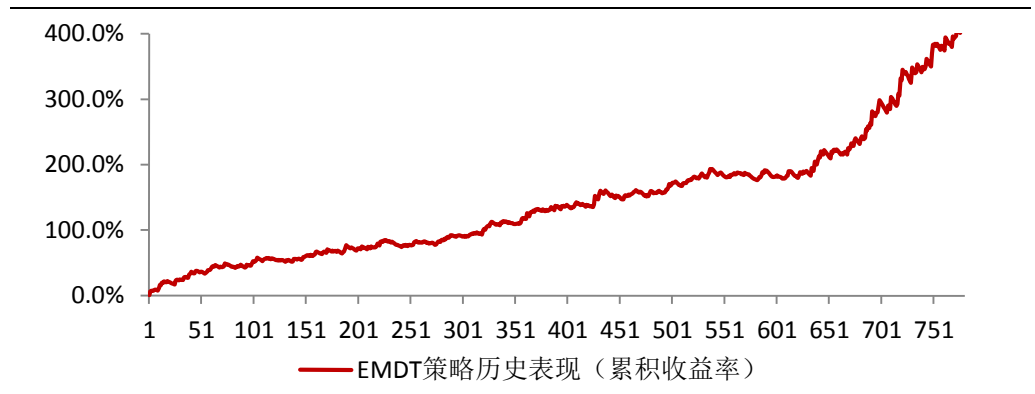
图 4: EMDT 策略历史表现 (自 2010 年 4 月 16 日起)
