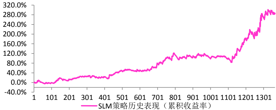
图 5: SLM 策略历史表现 (自 2010 年 4 月 16 日起)
