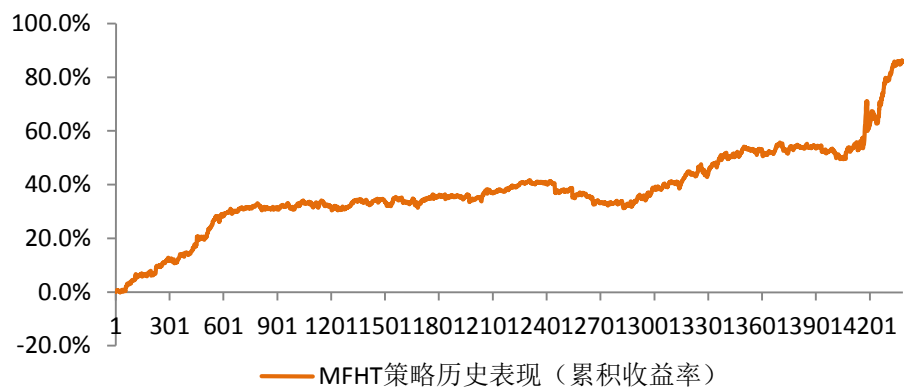
图 6: MFHT 策略历史表现 (自 2010 年 4 月 16 日起)
