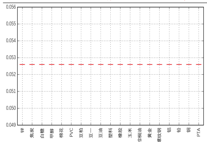
图表 29: 风险等权组合各资产的风险贡献度分布
