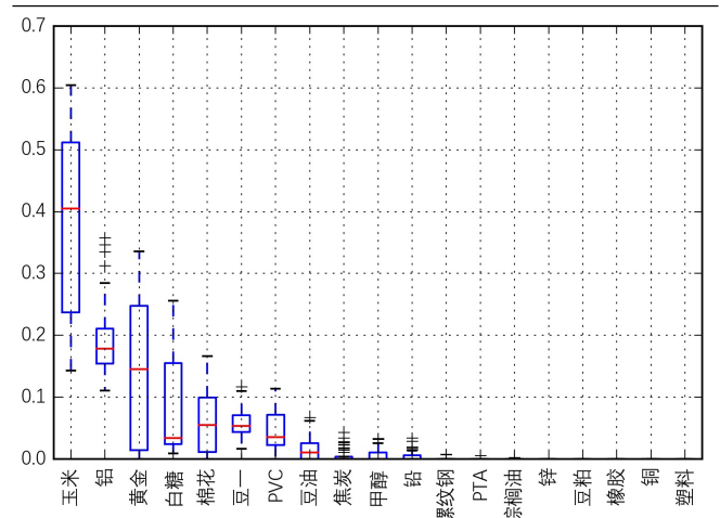
图表 21: 最小方差组合各资产的风险贡献度分布
