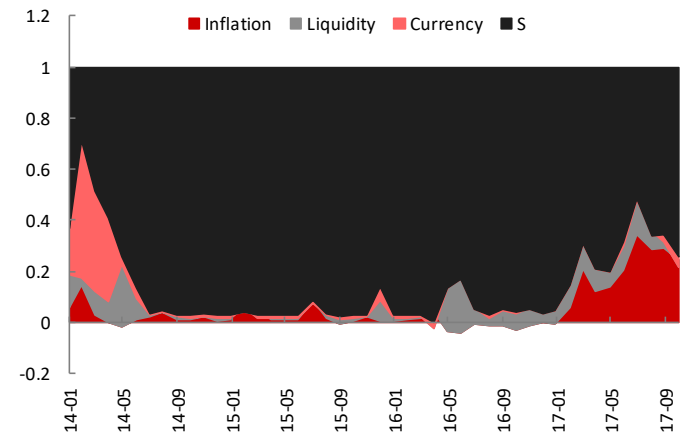
图表 47: S 因子全暴露组合的因子风险贡献度
