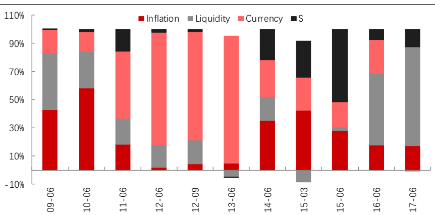
图表 14：南华商品综合指数基于风险因子的风险分解
