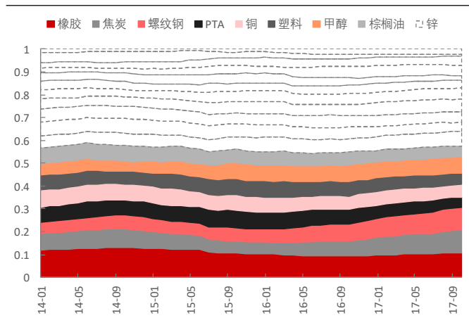
图表 8：等权重组合基于资产的风险分解
