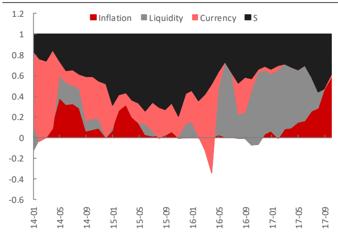
图表 26: 最大分散化组合基于风险因子的风险分解
