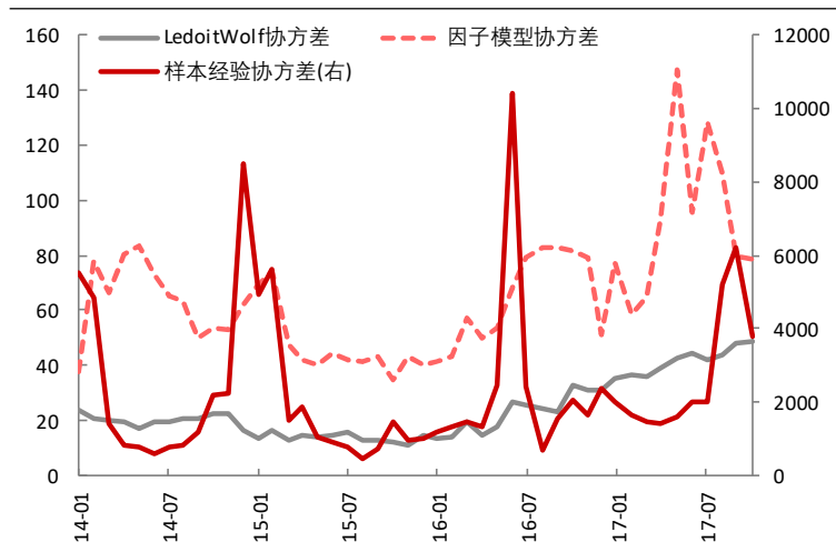
图表 7：三种协方差的条件数
