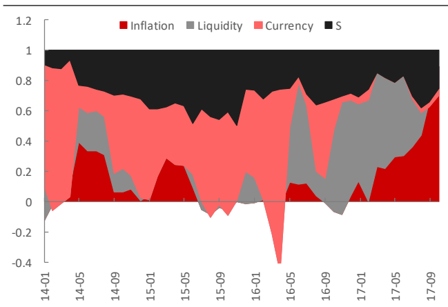
图表 30: 风险等权组合基于风险因子的风险分解
