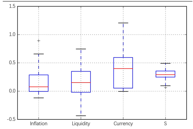
图表 31: 风险等权组合各因子的风险贡献度分布
