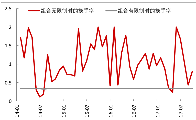
图表 36: 风险等权组合在有无限制时的换手率
