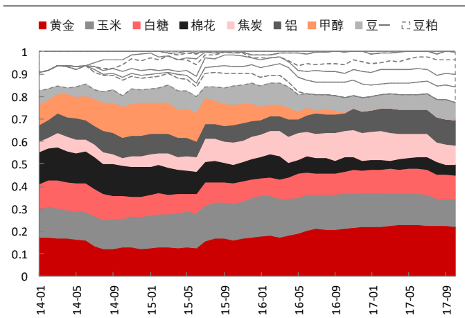
图表 24: 最大分散化组合基于资产的风险分解
