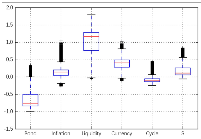
图表 3: 随机权重对应的 5 因子的风险贡献度
