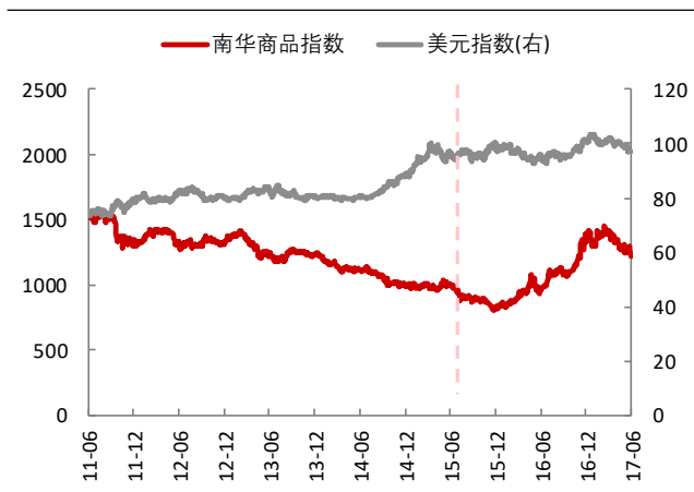
图表 15: 南华商品指数与美元指数
