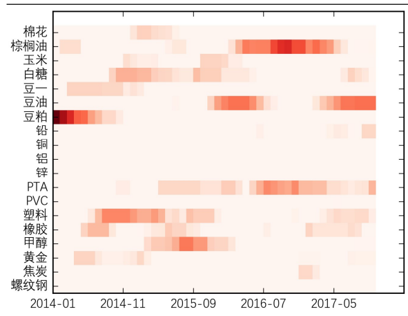
图表 42: Inflation 因子全暴露组合的资产权重分布
