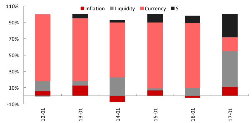
图表 19：监控中心商品指数基于风险因子的风险分解
