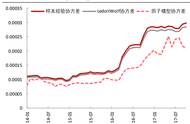
图表 6: 资产 i 与 j (i=j) 的平均协方差
