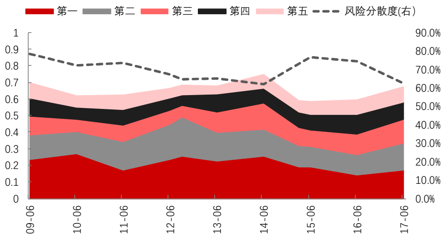
图表 13：南华商品综合指数基于资产的风险分解——累计风险贡献度
