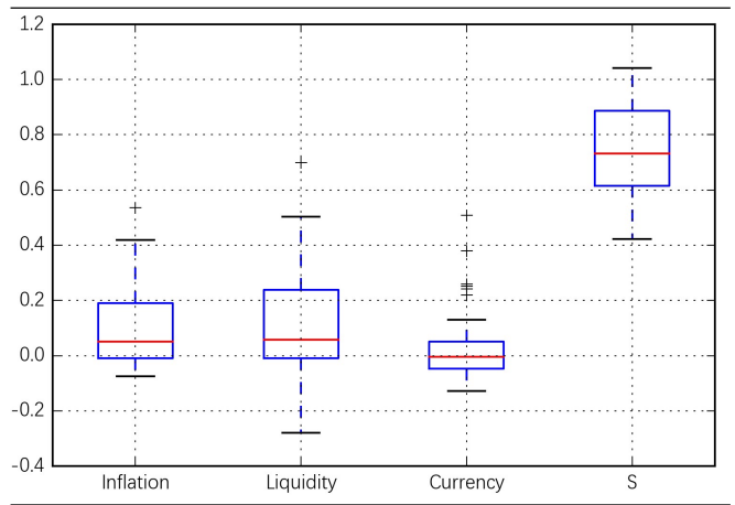
图表 23: 最小方差组合各因子的风险贡献度分布
