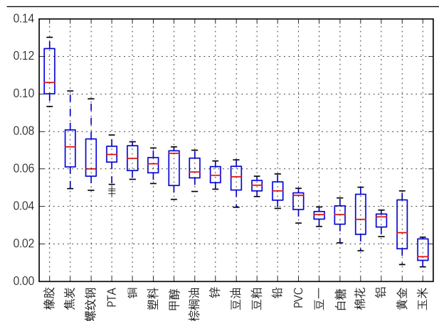
图表 9：等权重组合各资产的风险贡献度分布
