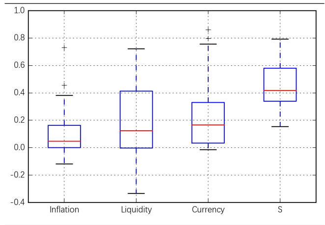
图表 27: 最大分散化组合各因子的风险贡献度分布
