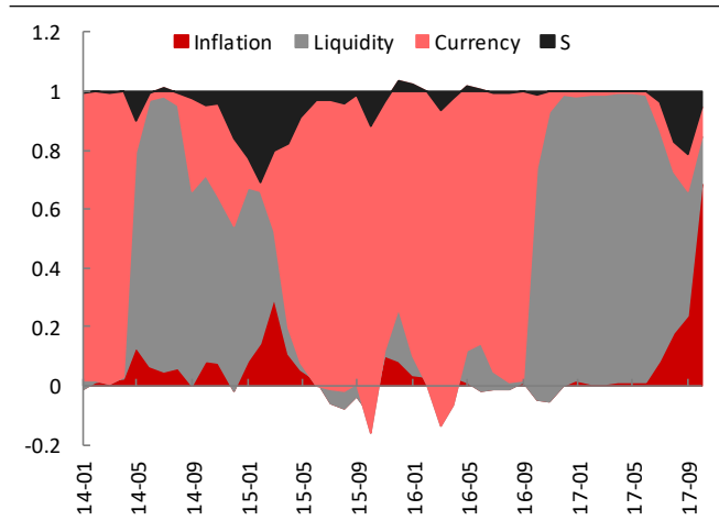
图表 52：滚动风险预算组合 1 的因子风险暴露度
