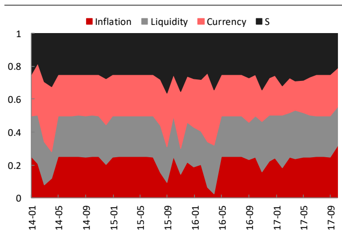
图表 34: 无限制时风险等权组合的因子风险贡献度
