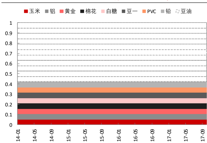
图表 28: 风险等权组合基于资产的风险分解
