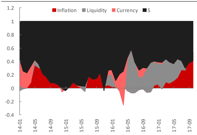
图表 22: 最小方差组合基于风险因子的风险分解
