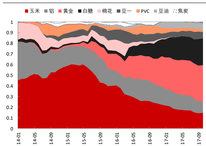
图表 20: 最小方差组合基于资产的风险分解
