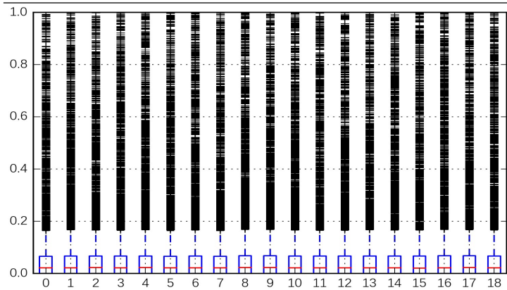
图表 2: 20000 组随机资产权重分布
