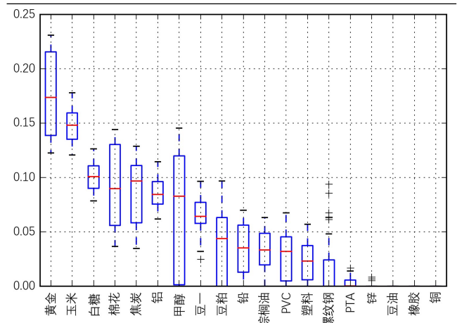
图表 25: 最大分散化组合各资产的风险贡献度分布
