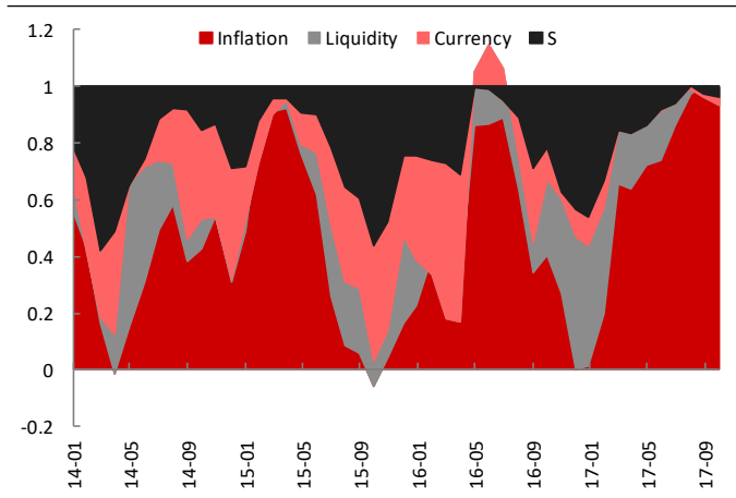
图表 41: Inflation 因子全暴露组合的因子风险贡献度
