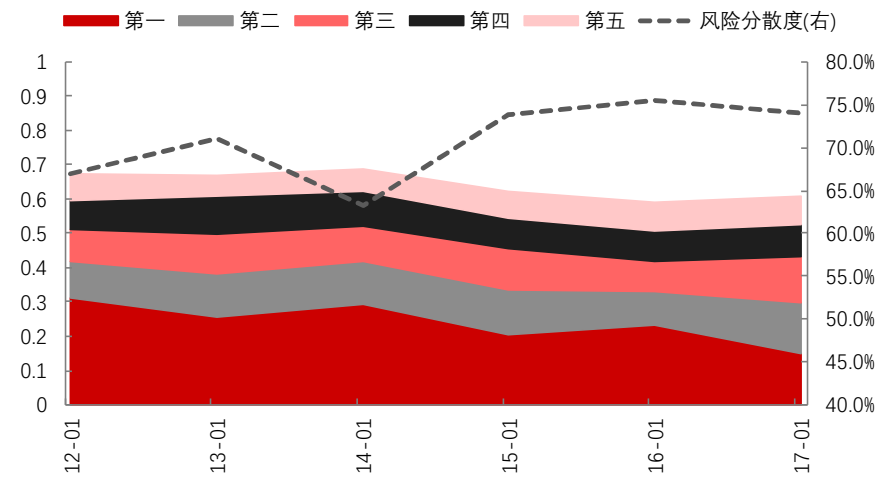
图表 18：监控中心商品指数基于资产的风险分解——累计风险贡献度
