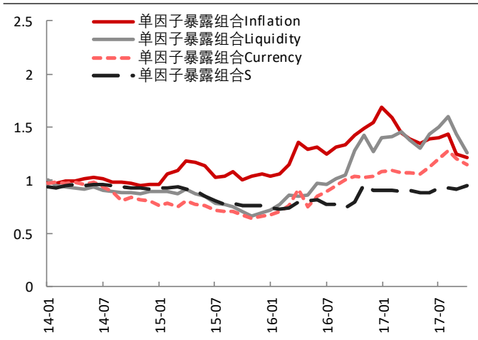
图表 49: 无换手限制时单因子全暴露组合的净值表现
