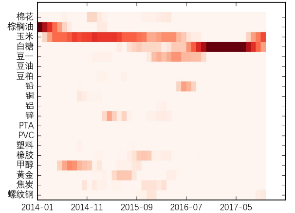
图表 48: S 因子全暴露组合的资产权重分布
