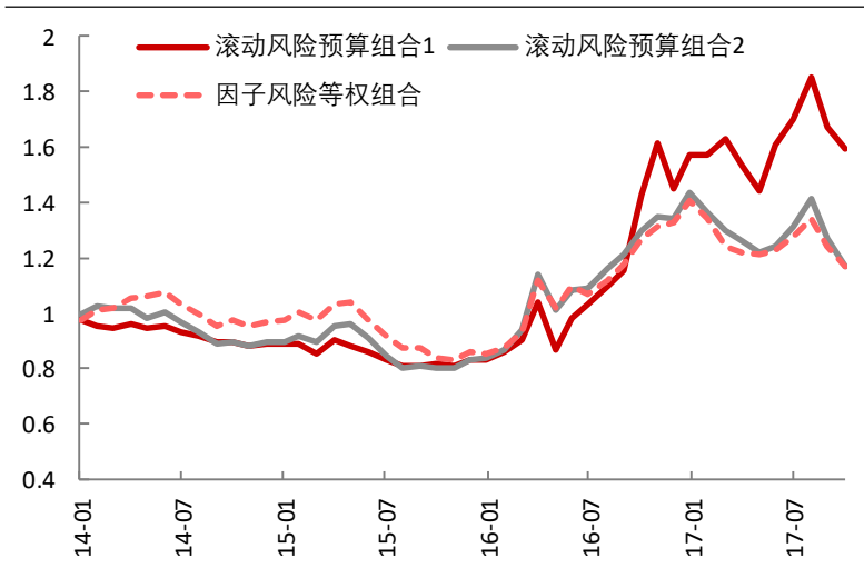
图表 54: 两种滚动风险预算组合与因子风险等权组合的净值对比
