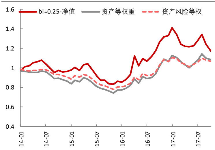
图表 39: 因子风险等权组合与资产等权重、资产风险等权组合的净值对比
