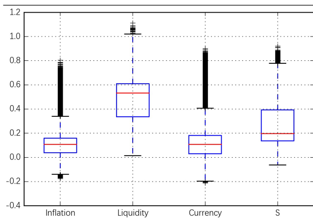
图表 4: 随机权重对应的 3 因子的风险贡献度
