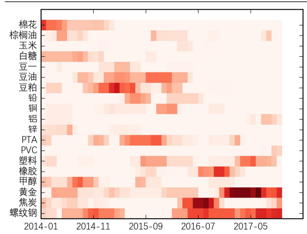
图表 46: Currency 因子全暴露组合的资产权重分布
