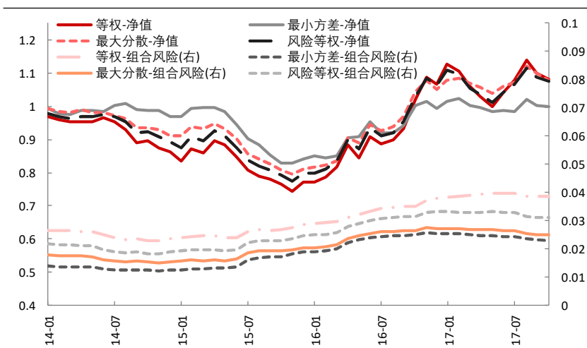
图表 32: 不同构建方式所得到的组合净值及组合风险的表现
