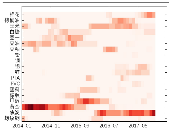
图表 44: Liquidity 因子全暴露组合的资产权重分布
