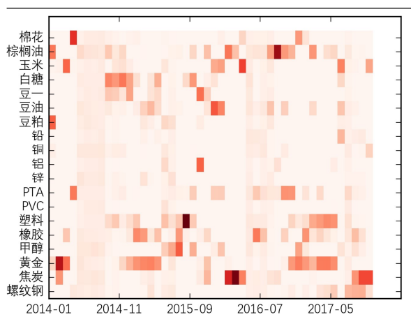
图表 35: 无限制时风险等权组合的资产权重分布
