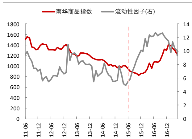
图表 16: 南华商品指数与流动性因子
