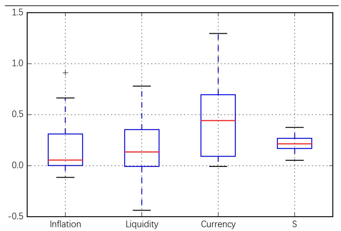
图表 11：等权重组合各因子的风险贡献度分布
