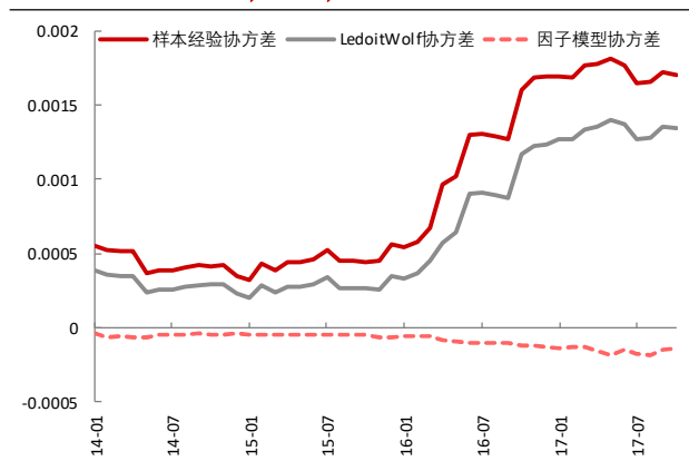
图表 5: 资产 i 与 j (i≠j) 的平均协方差
