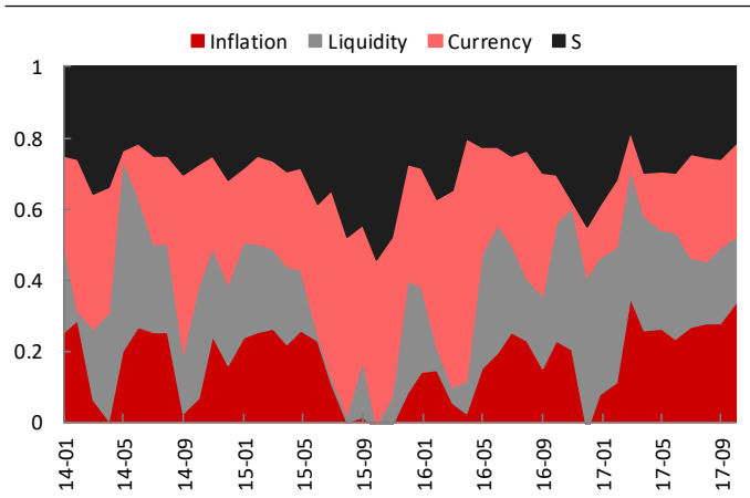
图表 37: 有限制时风险等权组合的因子风险贡献度
