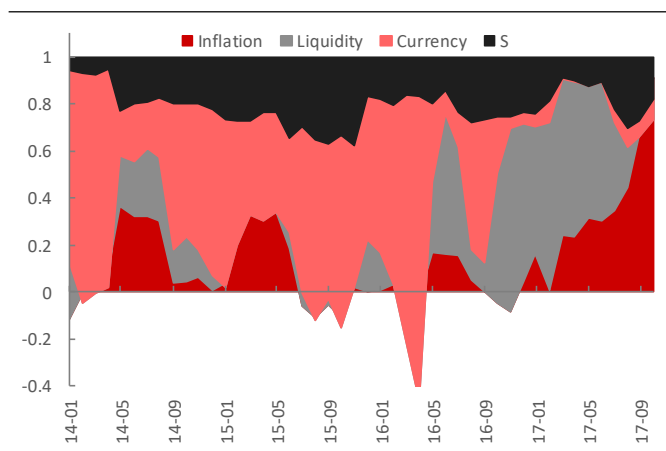
图表 10：等权重组合基于风险因子的风险分解
