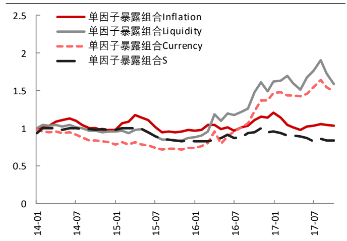
图表 50: 有换手限制时单因子全暴露组合的净值表现
