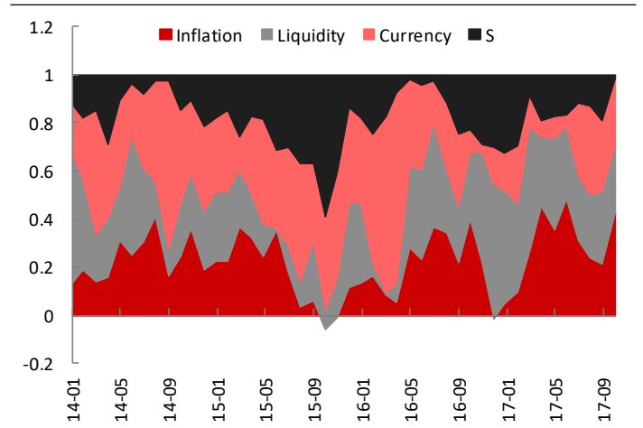
图表 53：滚动风险预算组合 2 的因子风险暴露度
