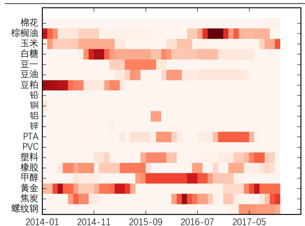
图表 38: 有限制时风险等权组合的资产权重分布
