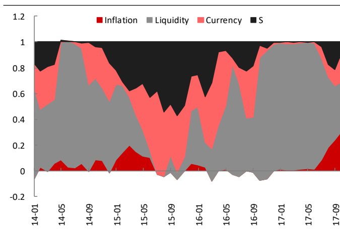
图表 43: Liquidity 因子全暴露组合的因子风险贡献度
