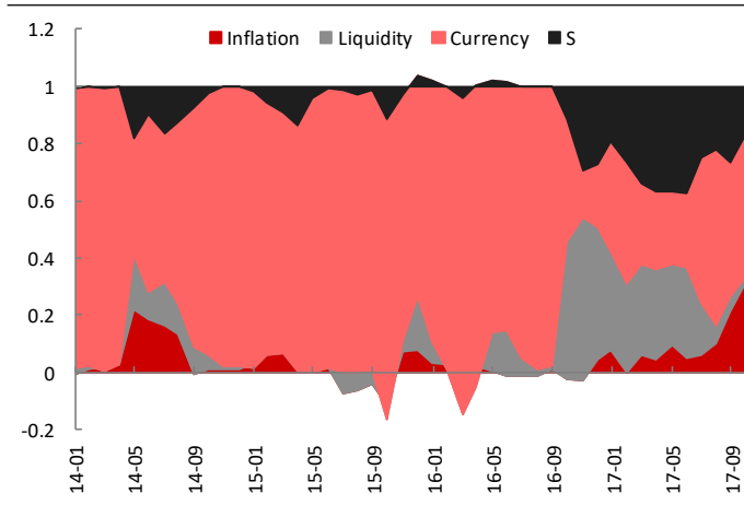
图表 45: Currency 因子全暴露组合的因子风险贡献度
