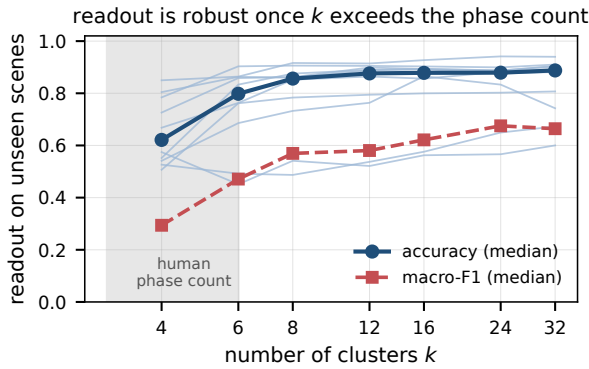
Figure 2: 군집 수 k 에 대한 판독 강건성. 사람 phase 수(3-6, 회색 대역)를 넘는 k \geq 8 에서 성능이 평평해진다(정확도 0.86-0.89). 열은 선 = instruction 10개.
