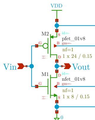
Gambar 1: Skematik desain inverter CMOS menggunakan PDK Skywater 130nm.
