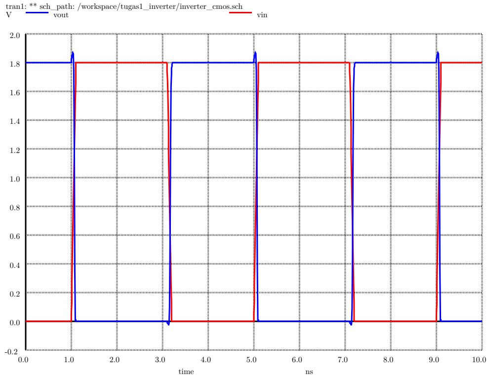
Gambar 2: Kurva simulasi transient tegangan input dan output terhadap waktu.
