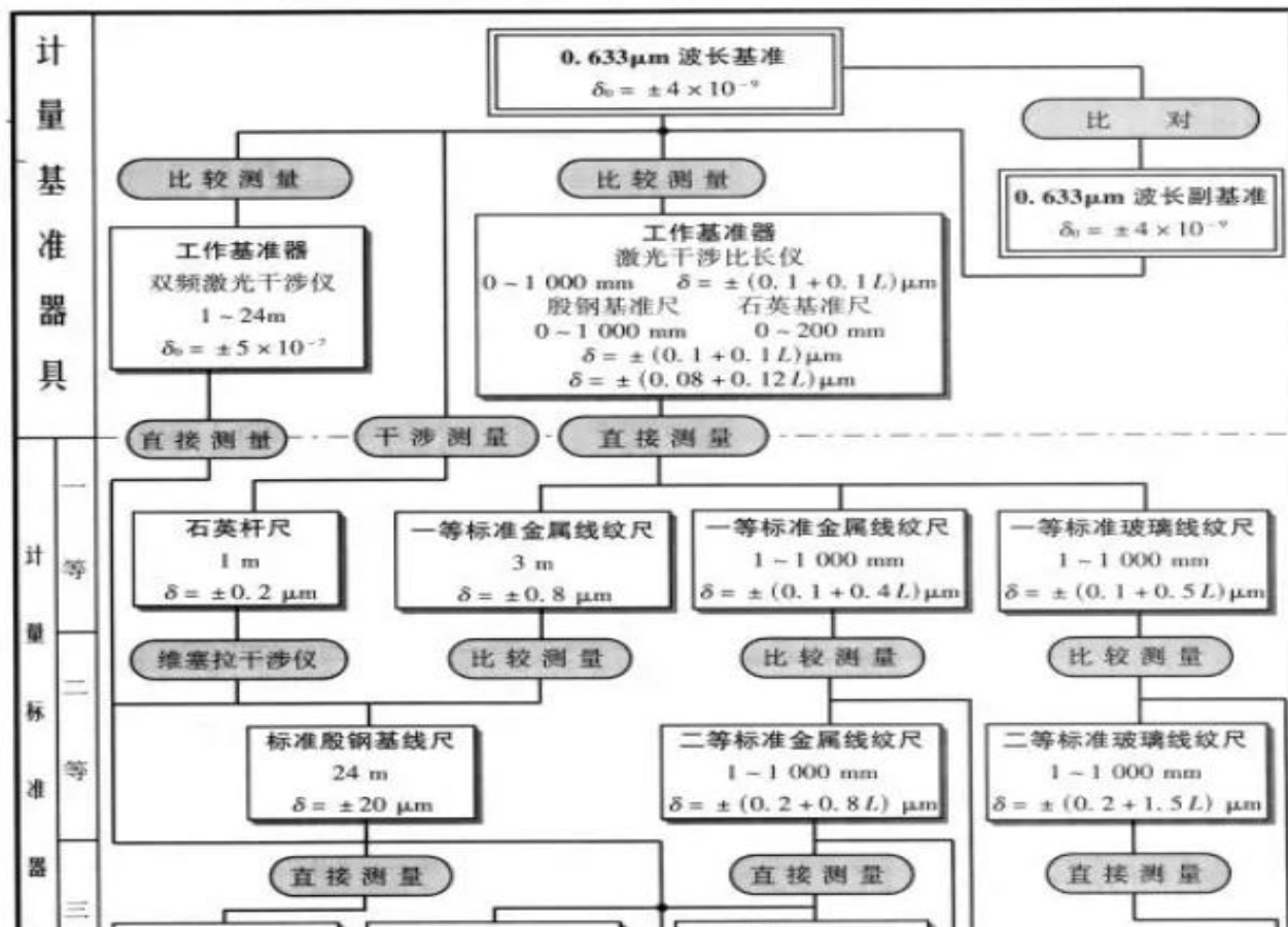
线纹计量器具检定系统框图
