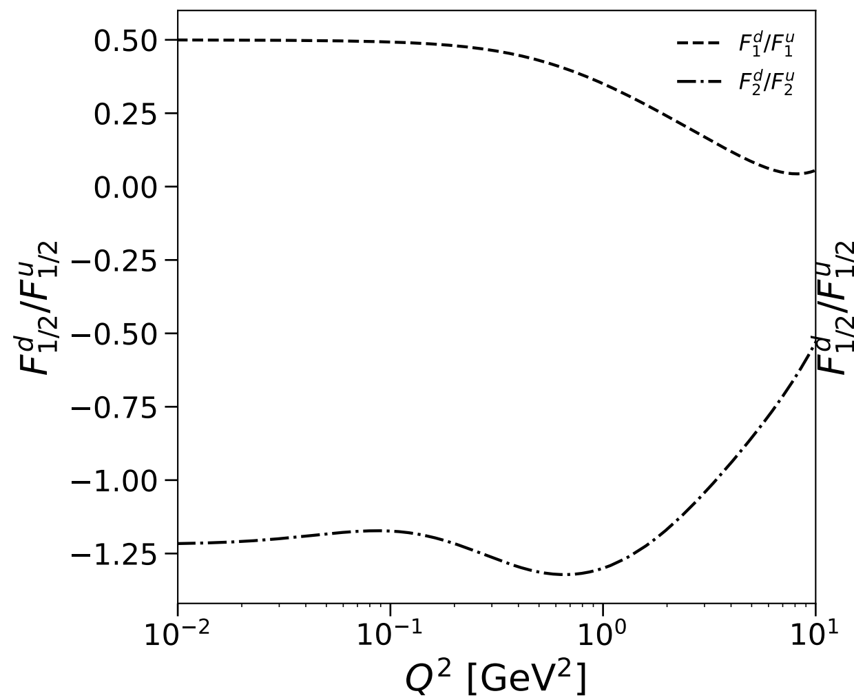
SBS Global Fit
