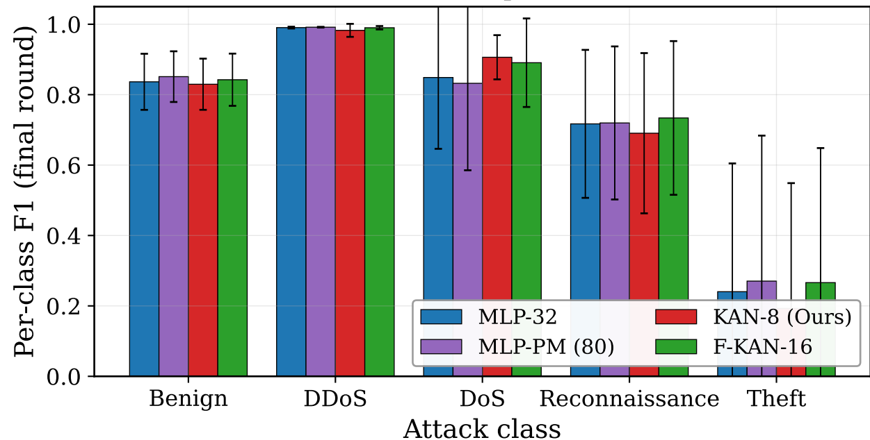
Multiclass — Dirichlet \alpha = 0.1 : per-class F1 (mean \pm 1 std)
