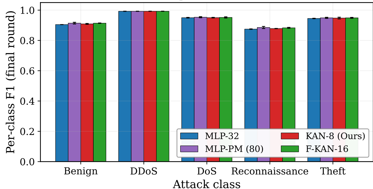
Multiclass — IID: per-class F1 (mean \pm 1 std)
