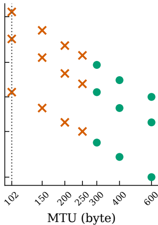
openssl
