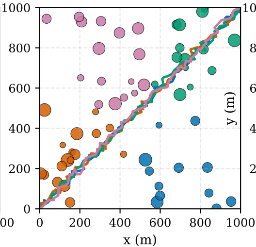
PSO
