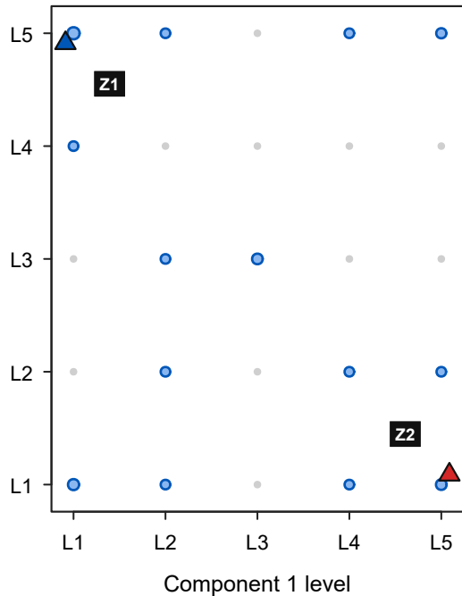
P-GP
