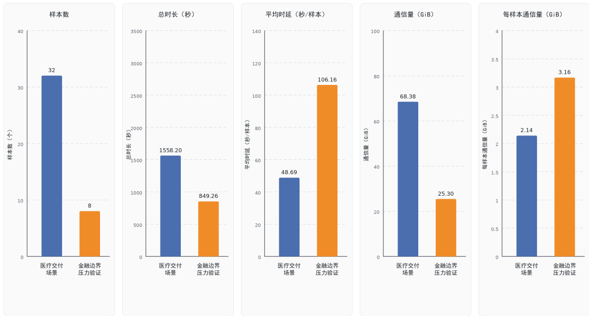
图 4-4 不同场景端到端性能与通信量统计
