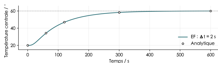
Figure 4. Température centrale ; pointillés : régime stationnaire à 60 ^\circ\text{C} .
