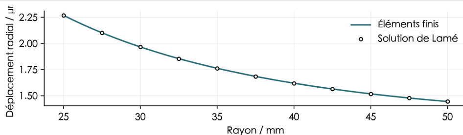
Figure 2. Déplacement radial dans l'épaisseur et solution de Lamé.
