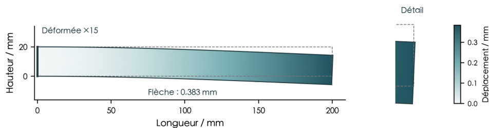
Figure 1. Déplacement de la poutre ; pointillés : forme initiale ; déformée \times 15 .
