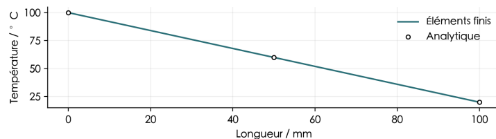
Figure 3. Température sur la ligne médiane horizontale.
