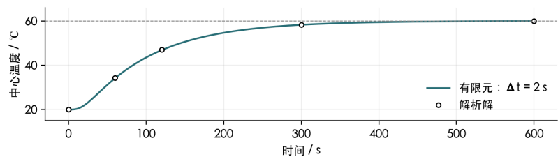
图 4 中心温度时间历程；虚线为稳态温度 60\text{ }^{\circ}\text{C} 。
