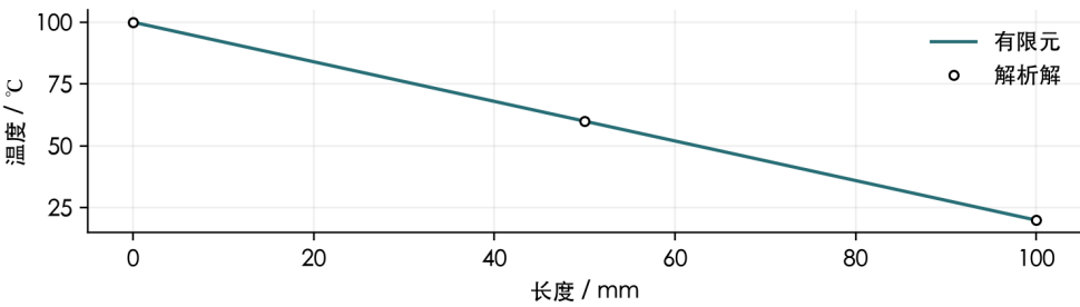
图 3 基准板沿水平中线的温度。
