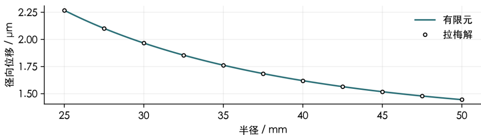
图 2 基准圆筒沿壁厚的径向位移与拉梅解。
