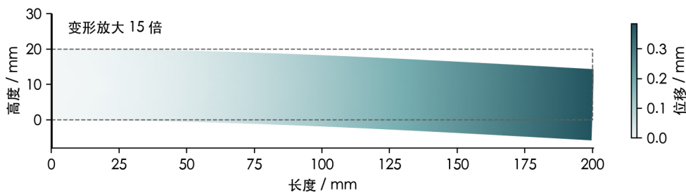
图 1 基准梁的位移；虚线为原形，变形放大 15 倍。
