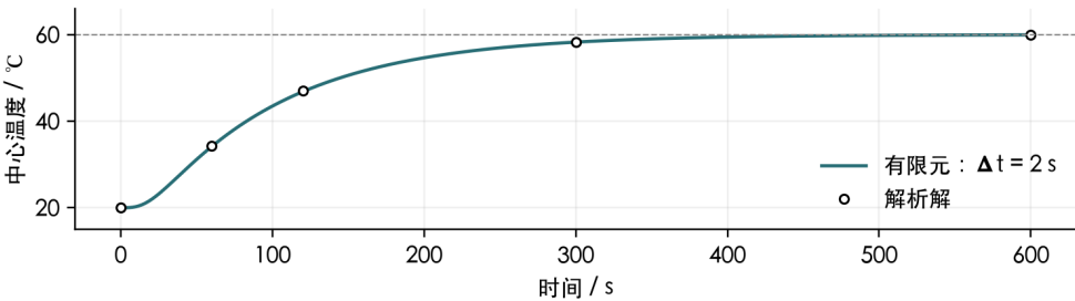
图 4 中心温度时间历程；虚线为稳态温度 60^\circ\text{C} 。
