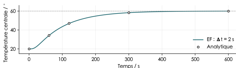
Figure 4. Température centrale ; pointillés : régime stationnaire à 60 °C.
