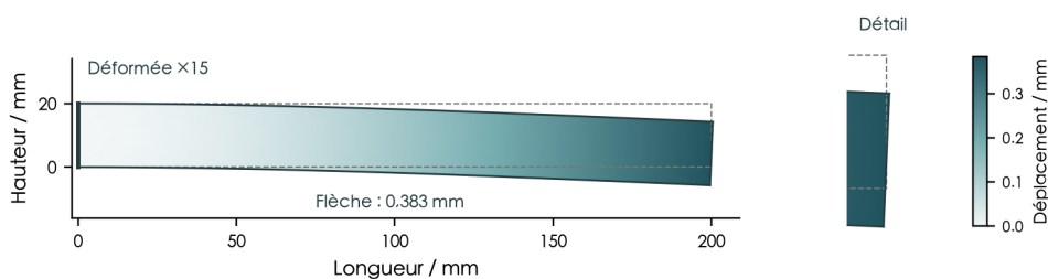
Figure 1. Déplacement de la poutre ; pointillés : forme initiale ; déformée \times 15 .
