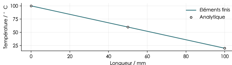
Figure 3. Température sur la ligne médiane horizontale.
