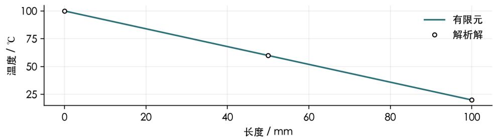
图 3 基准板沿水平中线的温度。
