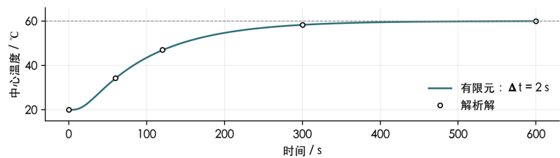
图 4 中心温度时间历程；虚线为稳态温度 60 °C。
