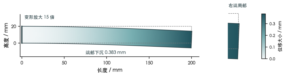
图 1 基准梁的位移：虚线为原形，变形放大 15 倍。
