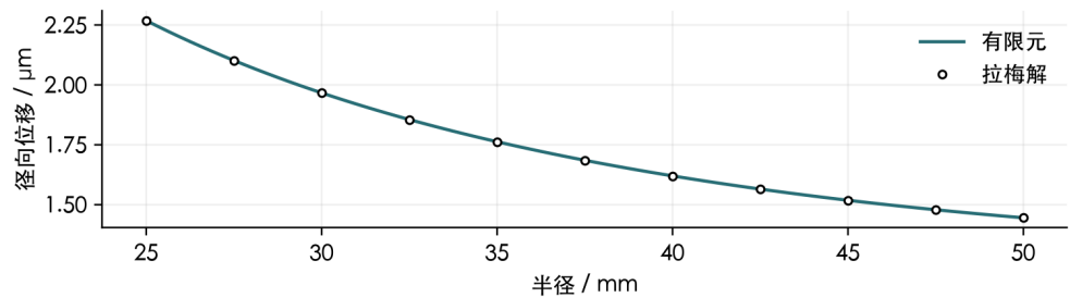
图 2 基准圆筒沿壁厚的径向位移与拉梅解。
