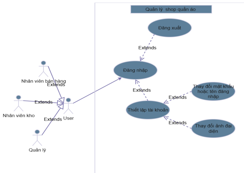
Hình 3.2 Sơ đồ Use Case đăng nhập.
