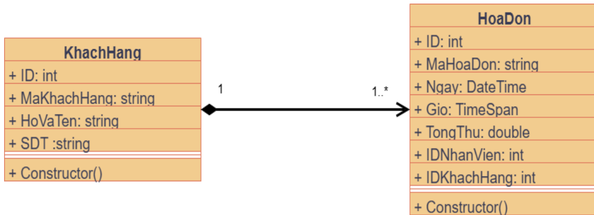
Hình 3.7 Class Diagram quan hệ giữa Hóa đơn và Khách hàng.
