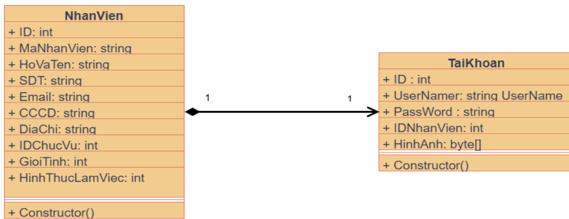
Hình 3.8 Class Diagram quan hệ giữa Nhân viên và Tài Khoản.
