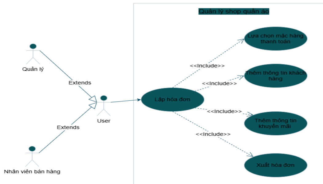
Hình 3.3 Sơ đồ Use Case Lập hóa đơn.
