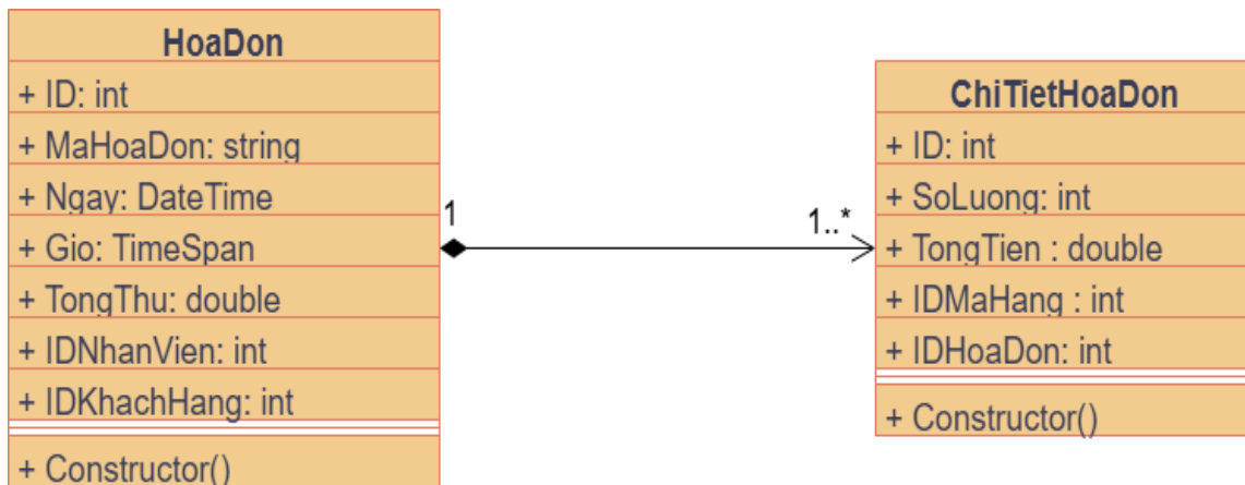
Hình 3.5 Class Diagram quan hệ giữa Hóa đơn và Chi tiết hóa đơn.
