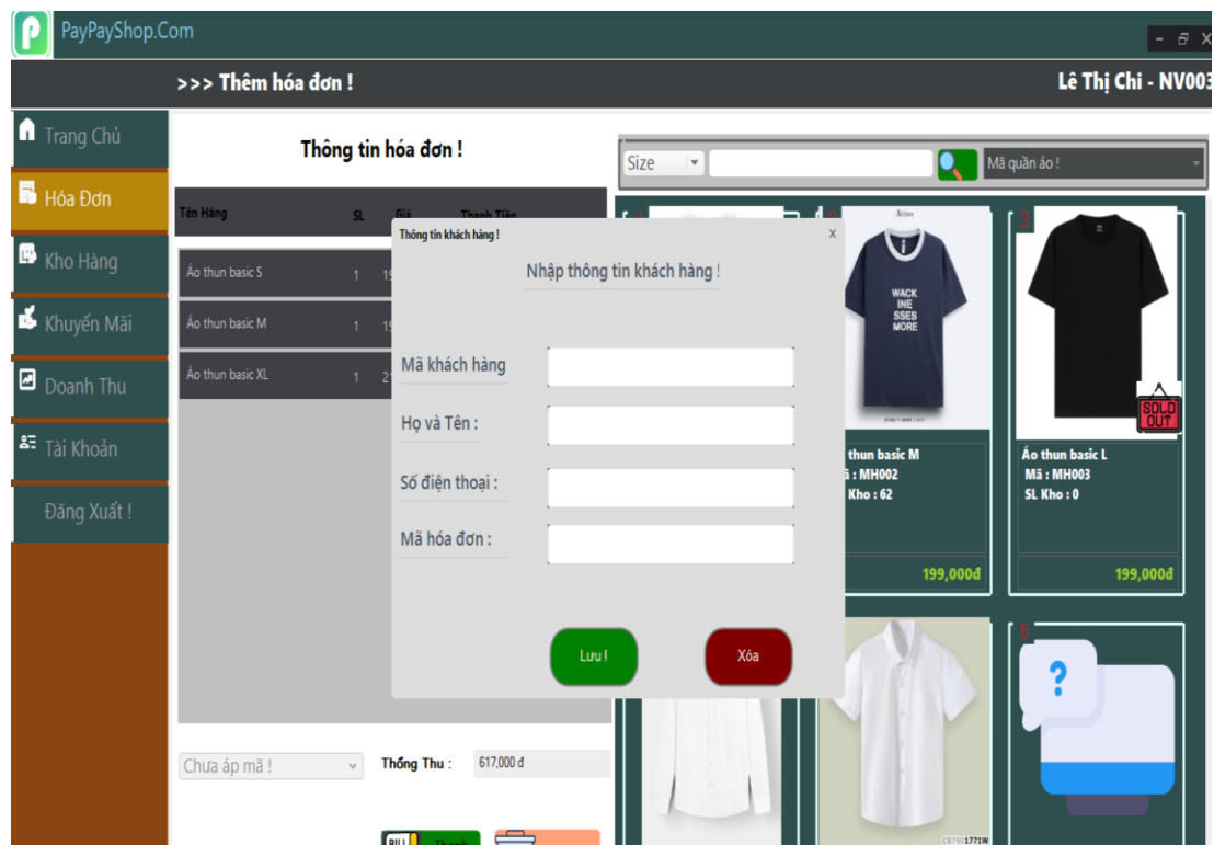
Hình 4.12 Giao diện Hóa Đơn Nút thanh toán.
