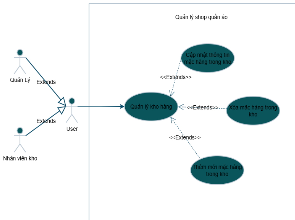
Hình 3.4 Sơ đồ Use Case Quản lý kho hàng.
