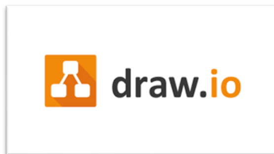
Hình 2.4 Draw.io
