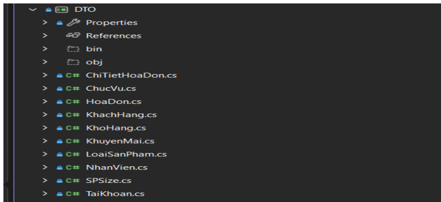
Hình 4.2 Project DTO.
