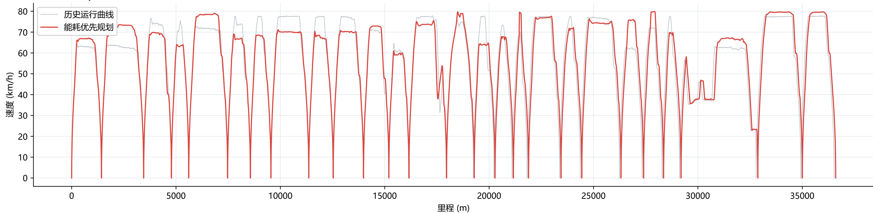
b 速度-里程 | 规划里程 36.602 km
