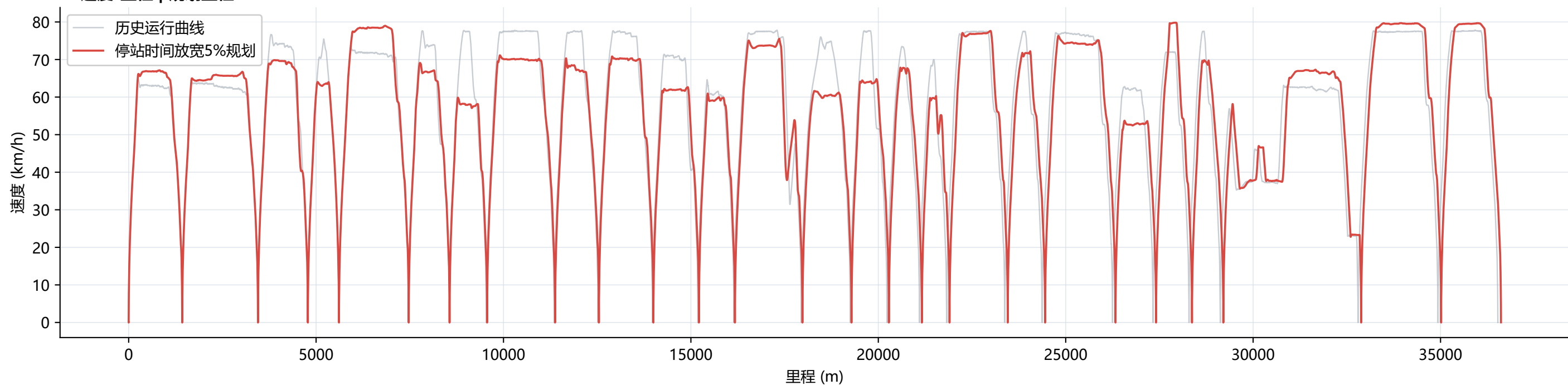
b 速度-里程 | 规划里程 36.613 km
