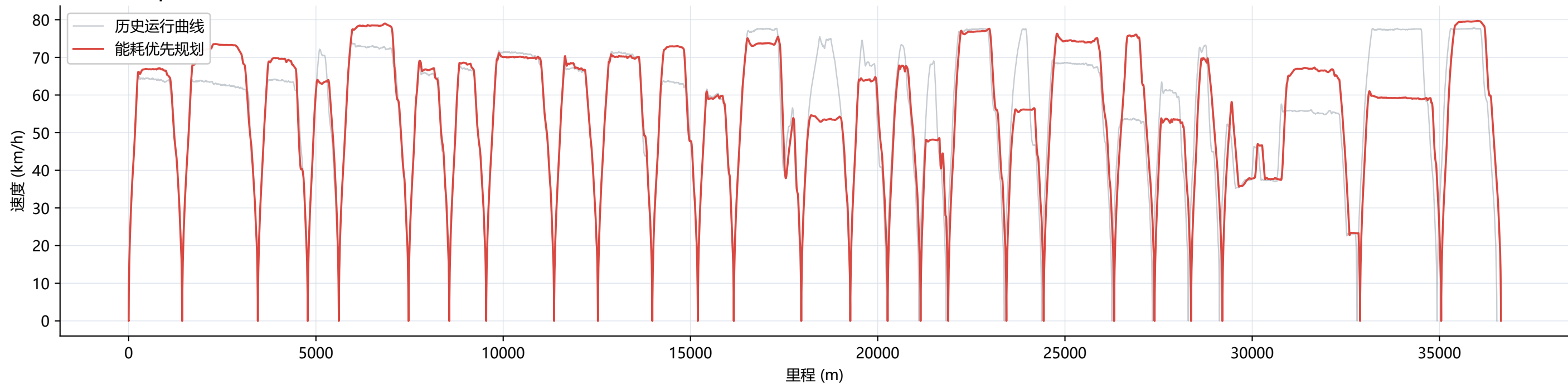
b 速度-里程 | 规划里程 36.643 km
