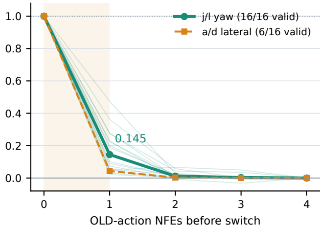
(b) minWM Wan2.1 Action2V
