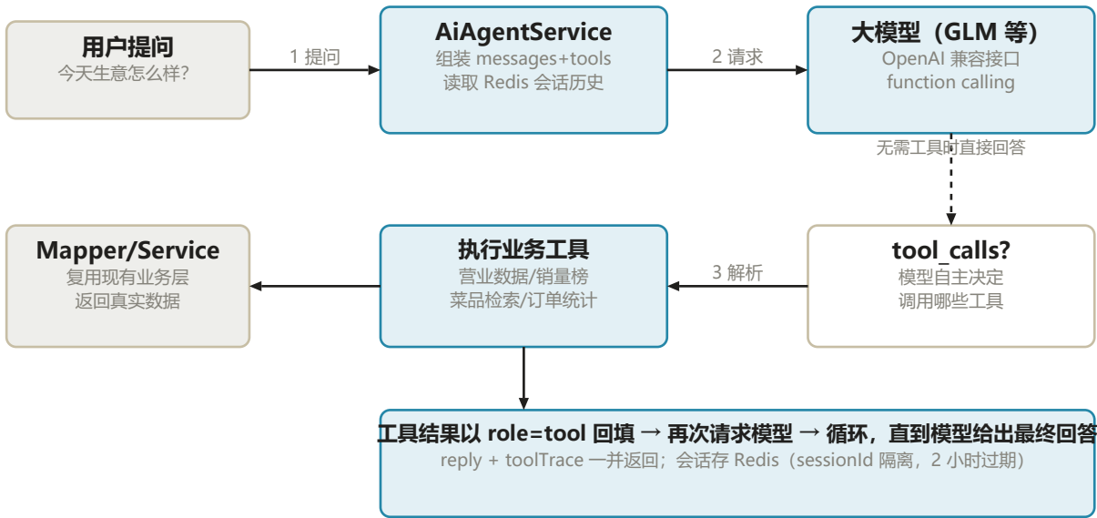
图 5-1 Tool-Calling Agent 循环（ReAct 思想）
