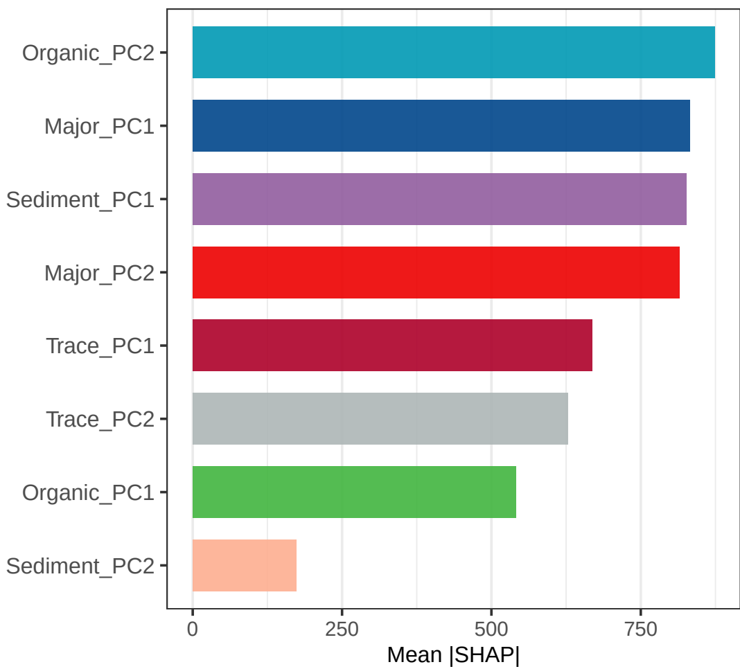
Rotaliida (RF)
