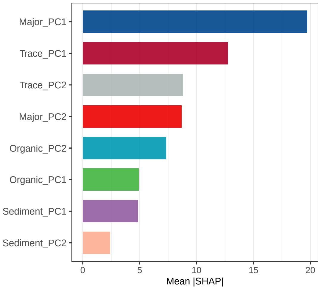
Rotaliida (RF)
