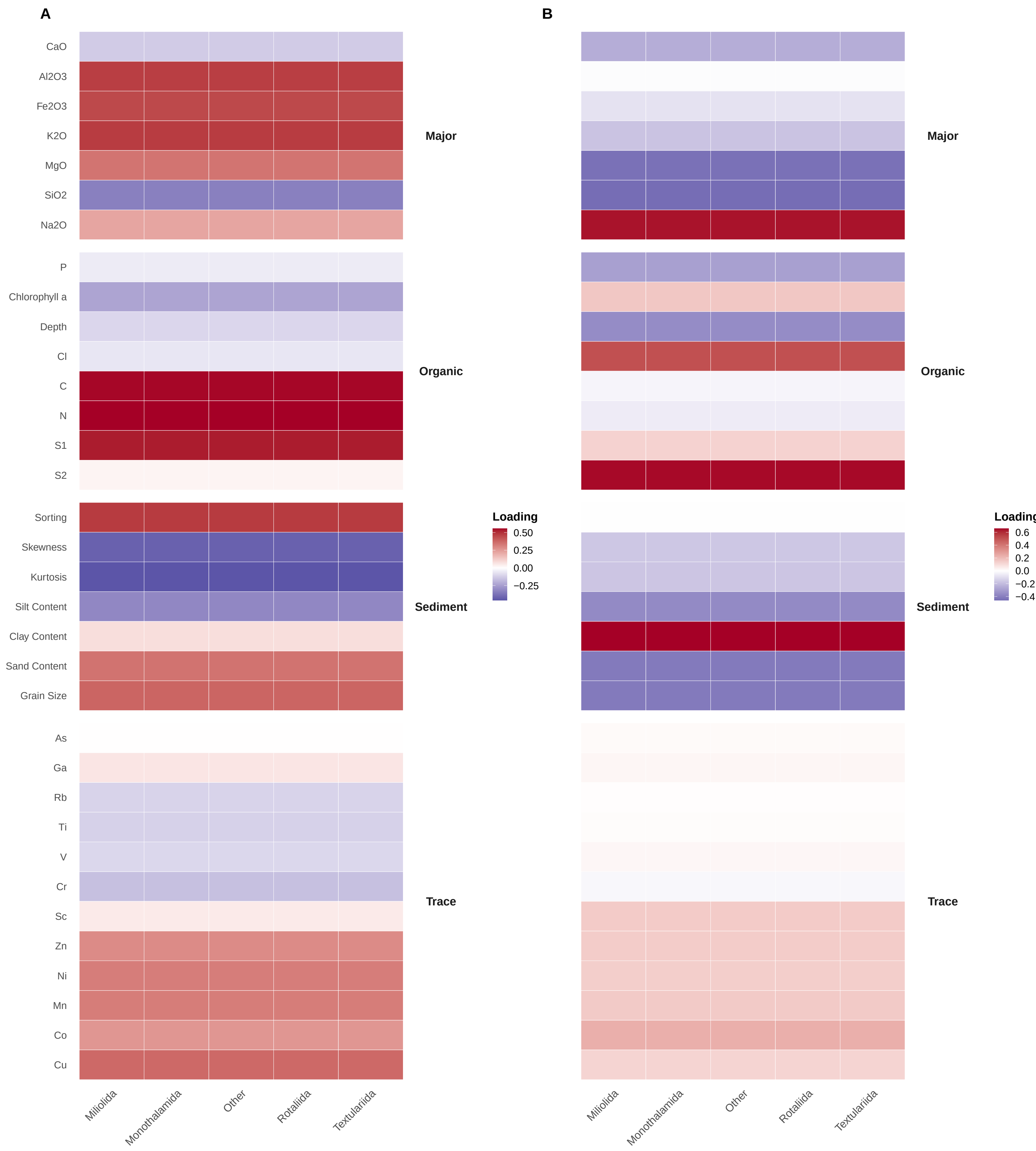
PCA Loadings (PC1 vs PC2)
