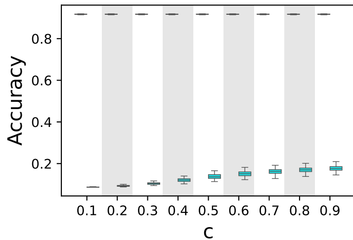
\eta_1(x) vs \xi_1(x)
