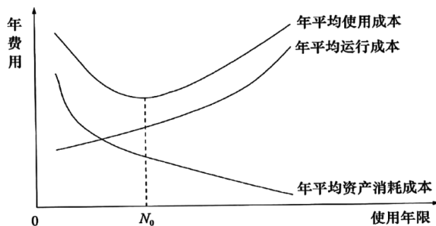
图 4.2-1 设备年费用及经济寿命
