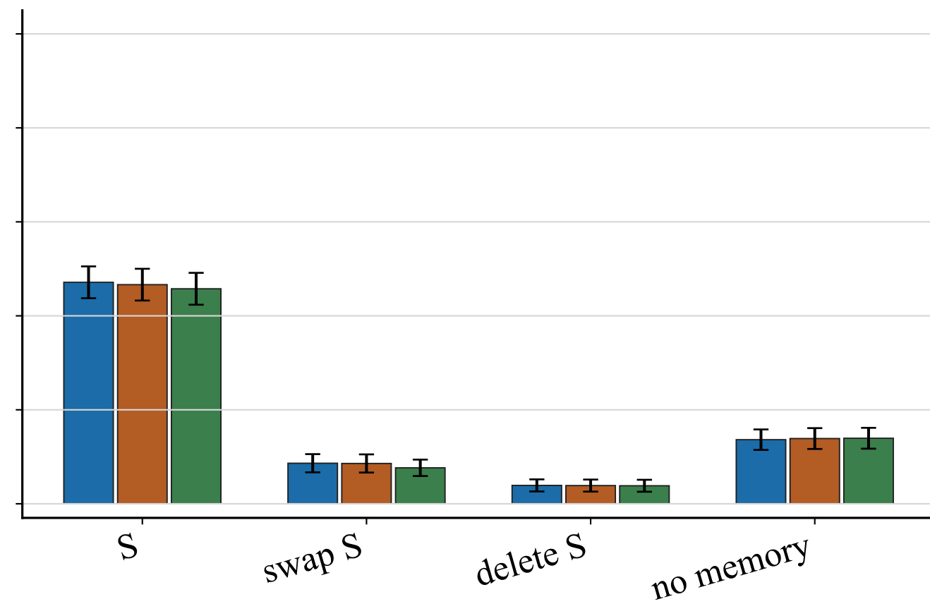
LoCoMo
