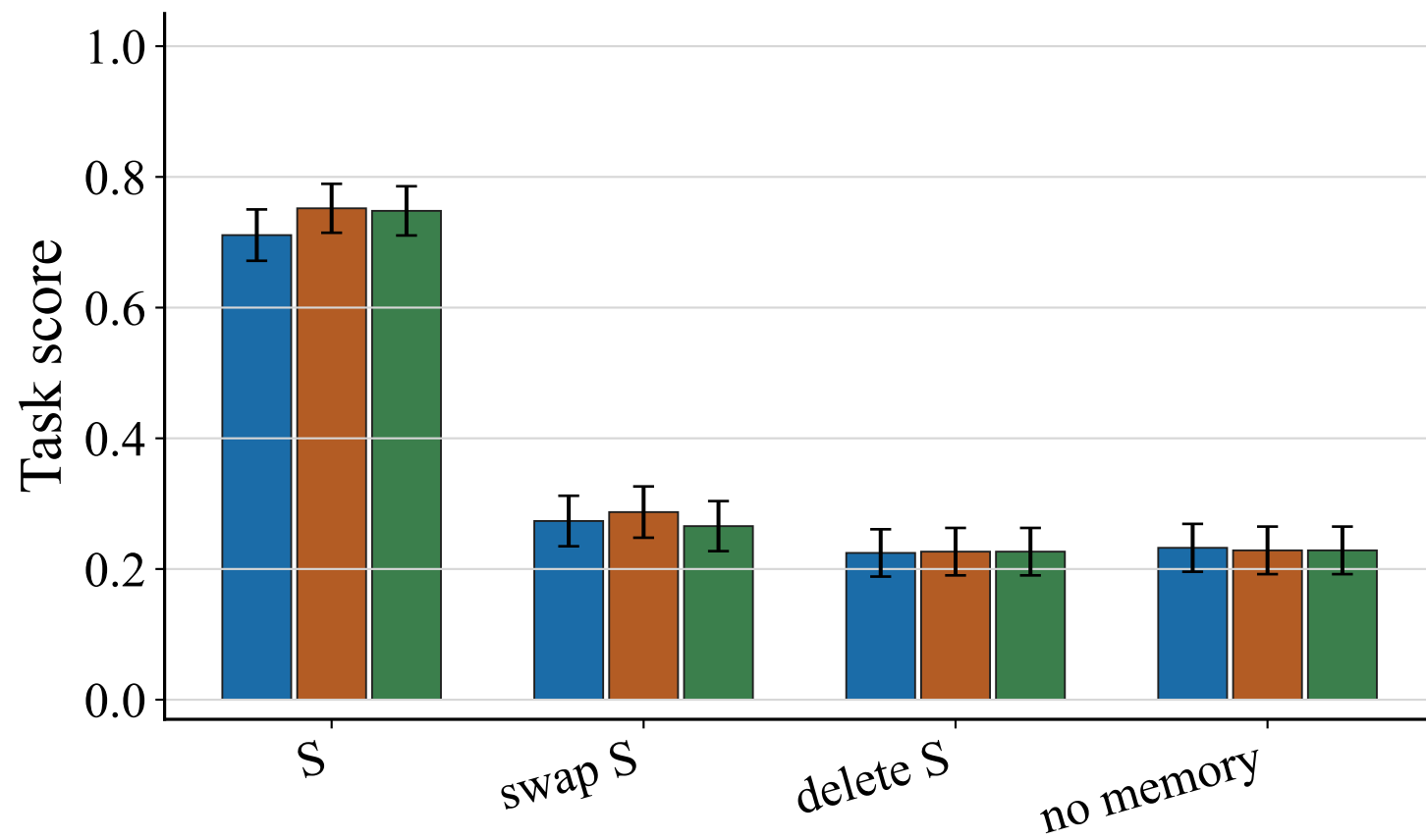
PersonaMem-v2
