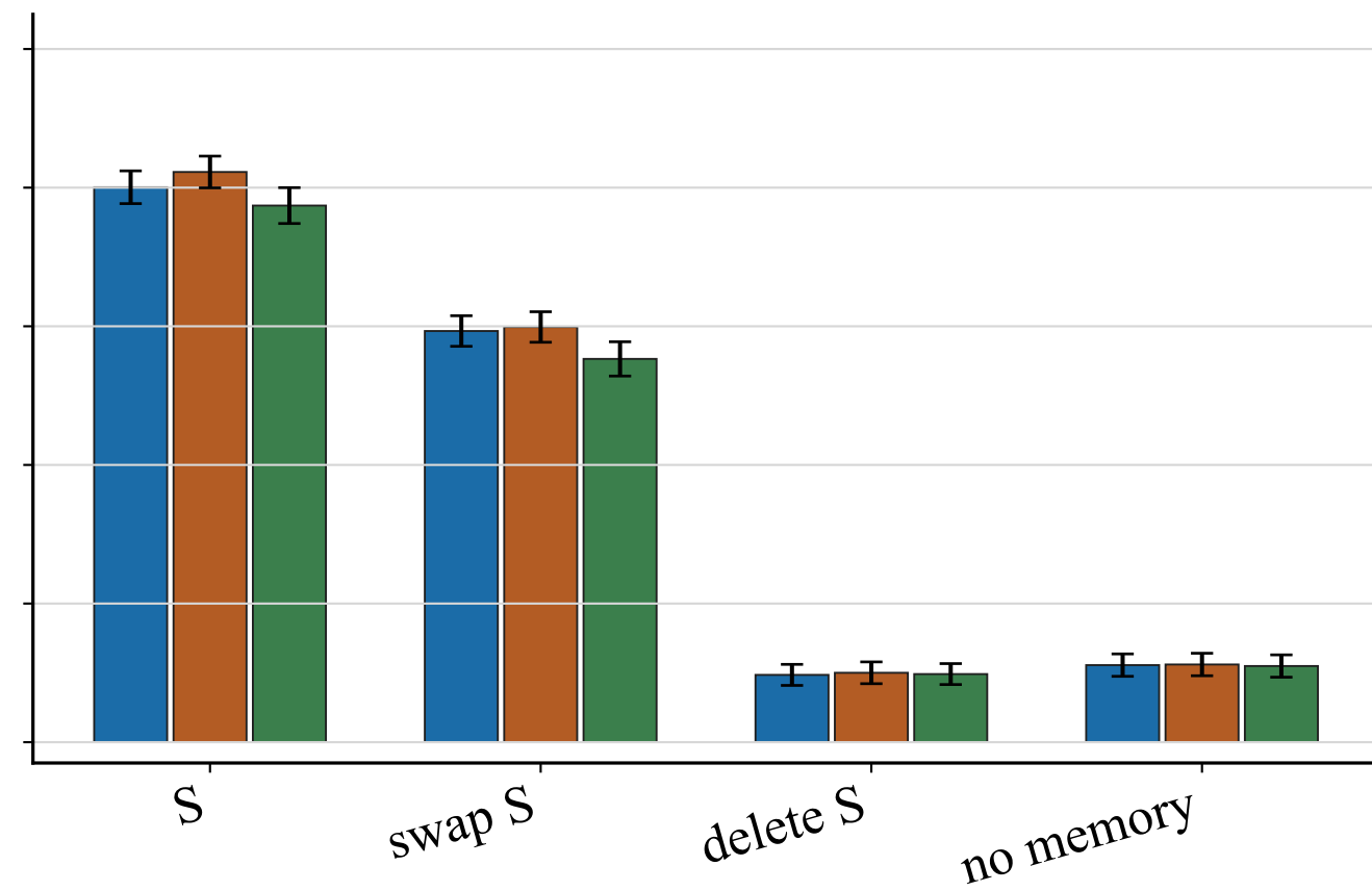
PersonaLens
