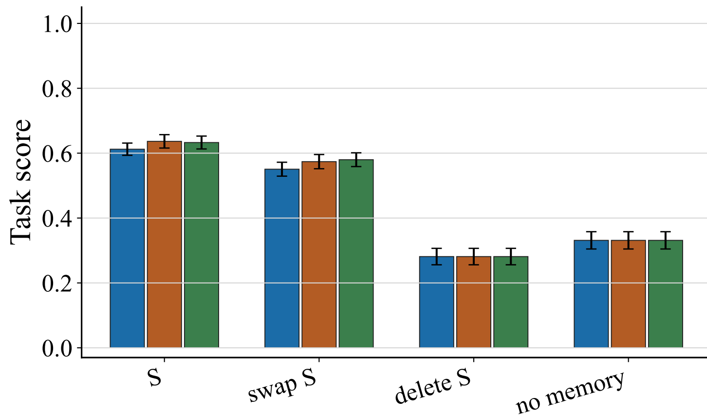
ETAPP
