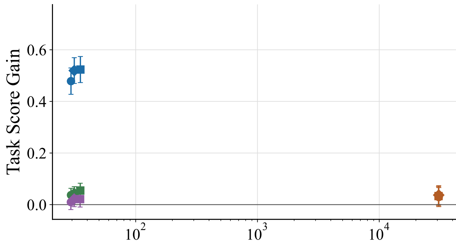
PersonaMem-v2
