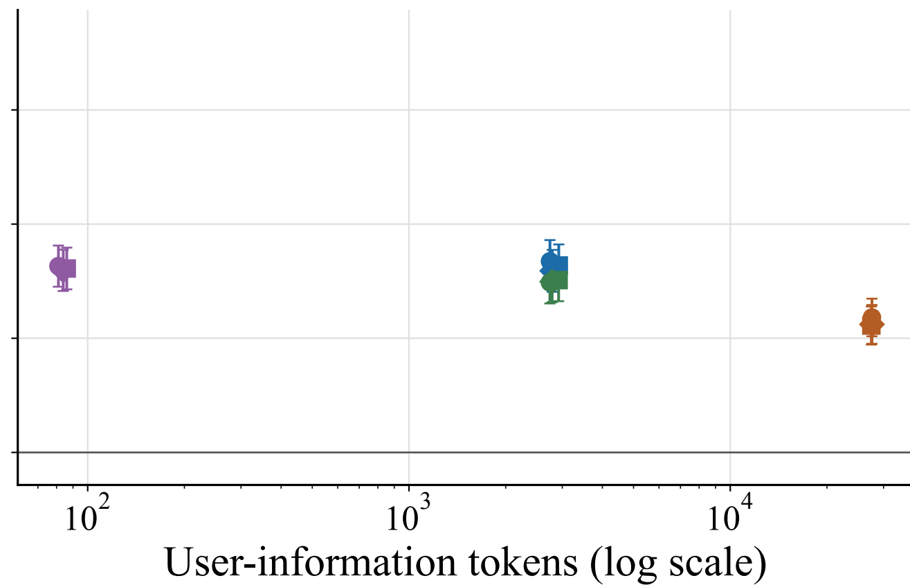
LoCoMo
