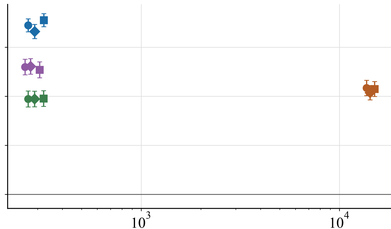
PersonaLens
