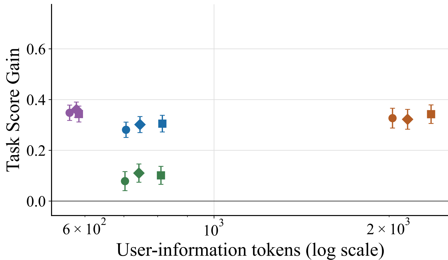
ETAPP
