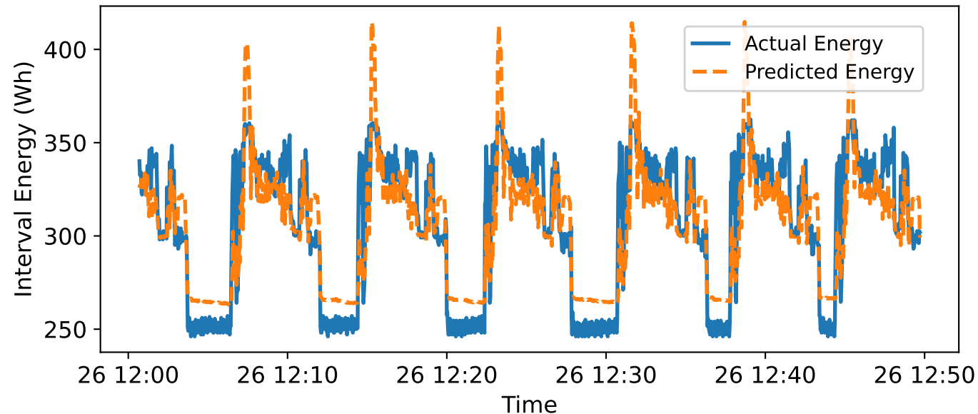
Actual vs. Predicted Interval energy
