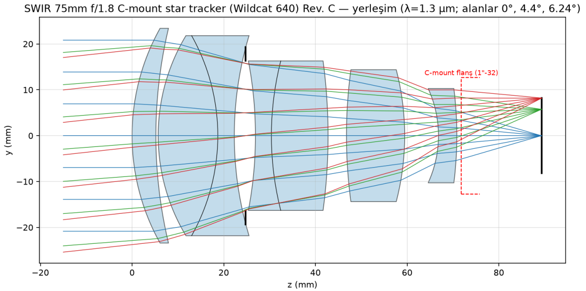
Şekil 1. Optik yerleşim, \lambda = 1,3 \mu\text{m} ; 0^\circ, 4,4^\circ ve 6,24^\circ alanlar. Kırmızı kesikli çizgi C-mount flanş düzlemi ve 1" diş açıklığıdır; alan düzleştirici flanşın hemen önünde, diş içinde durur.
