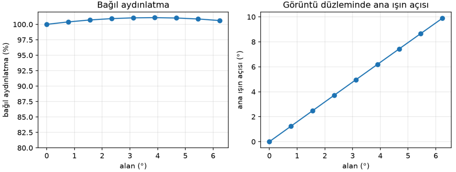
Şekil 12. Bağıl aydınlatma (yön kosinüsü uzayında çıkış konisi alanı, eksene göre) ve görüntü düzleminde ana ışın açısı.
