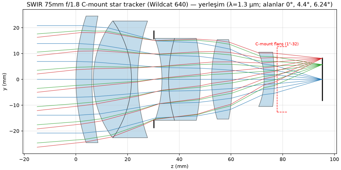
Şekil 1. Optik yerleşim, \lambda = 1,3 \mu\text{m} ; 0^\circ, 4,4^\circ ve 6,24^\circ alanlar. Kırmızı kesikli çizgi C-mount flanş düzlemi ve 1" dış açıklığıdır; alan düzleştirici flanşın hemen önünde, dış içinde durur.
