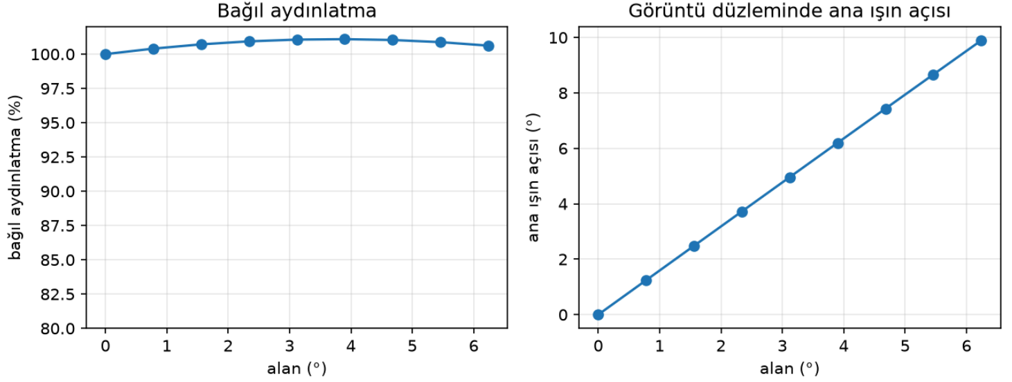
Şekil 10. Bağıl aydınlatma (yön kosinüsü uzayında çıkış konisi alanı, eksene göre) ve görüntü düzleminde ana ışın açısı.
