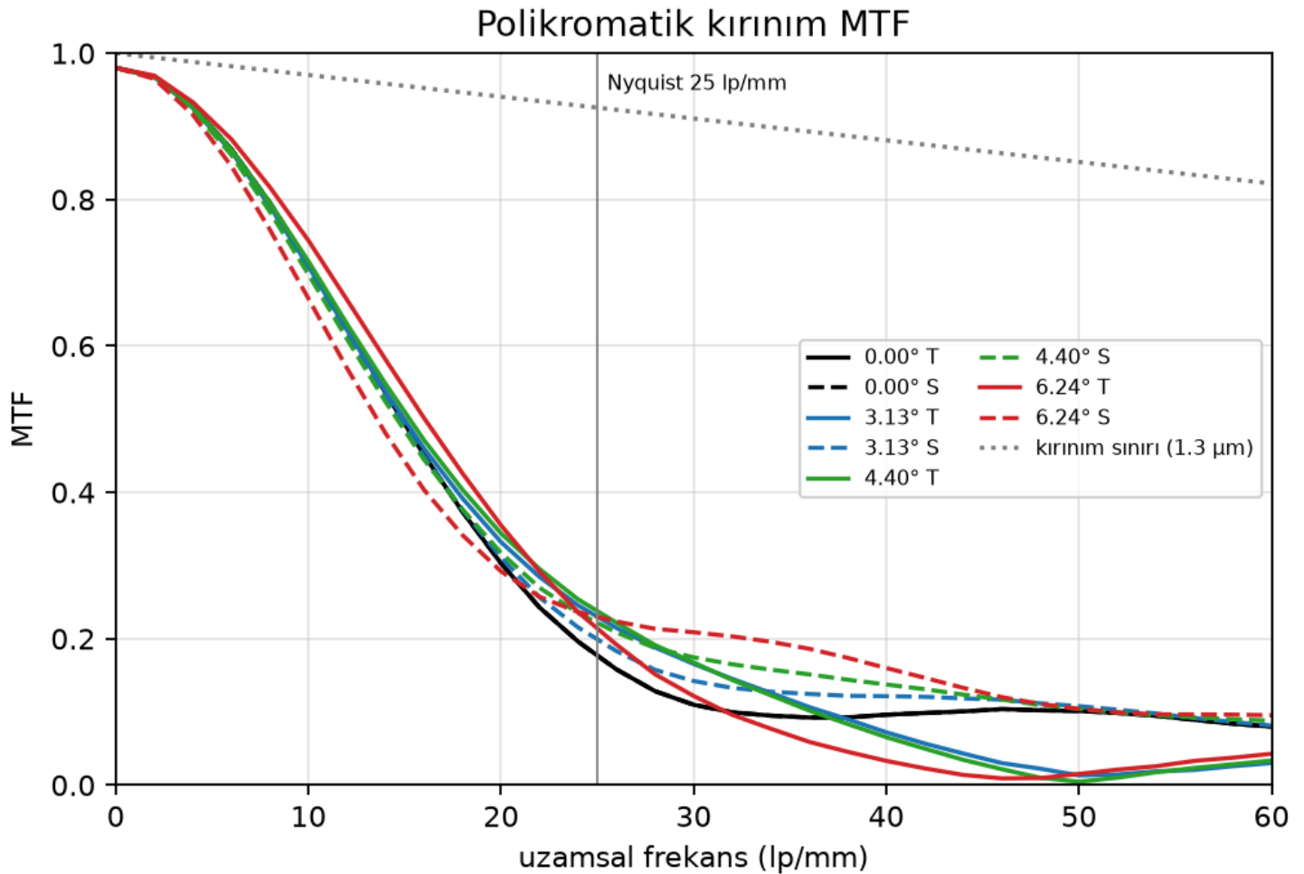
Şekil 7. Polikromatik kırınım MTF'si, tanjantsal (düz) ve sagital (kesikli), 4 alan; gri noktalı çizgi 1,3 \mu\text{m} kırınım sınırı, düşey çizgi 25 lp/mm Nyquist.
