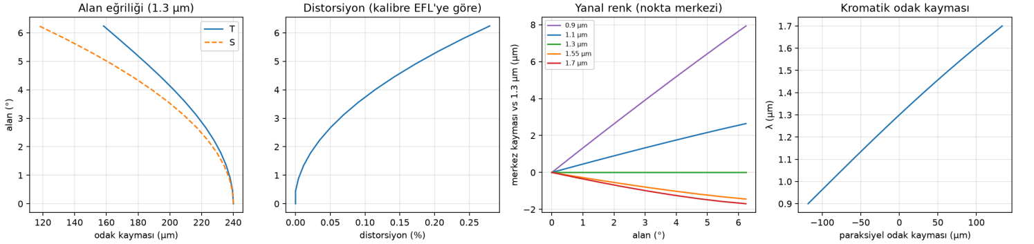
Şekil 9. Soldan sağa: tanjantsal/sagital paraksiyel odak konumu (görüntü düzlemine göre; nominal düzlem paraksiyel odağın önündedir), kalibre EFL'ye göre distorsiyon, dalga boyuna göre nokta merkezi kayması (yanal renk), paraksiyel kromatik odak kayması.
