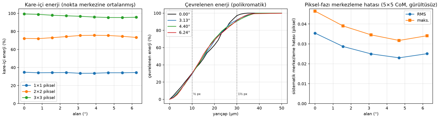
Şekil 5. Soldan sağa: kare-içi enerji ( 1 \times 1 , 2 \times 2 , 3 \times 3 px) alan boyunca; çevrelenen enerji profili (tüm alanlar üst üste biner); piksel-fazı merkezleme hatası RMS ve maksimum.
