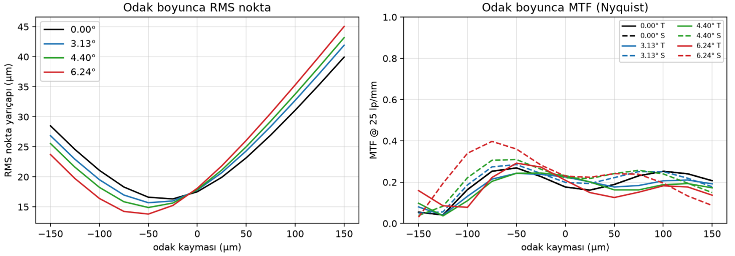
Şekil 6. Odak boyunca RMS nokta yarıçapı (sol) ve 25 lp/mm'de MTF (sağ). RMS minimumu bilinçli olarak nominal düzlemin \sim 50 \mu\text{m} önündedir; nominal düzlem, alan boyunca tekdüzelik ve odak duyarsızlığı için seçilmiştir.
