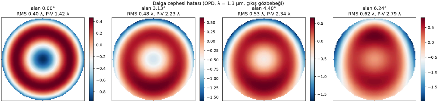
Şekil 8. Çıkış gözbebeğinde OPD haritaları, \lambda = 1,3 \mu\text{m} (birim: dalga).
