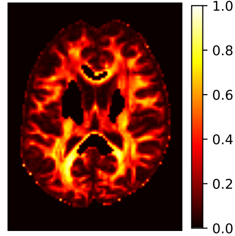
DIPY FA
