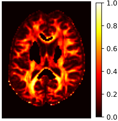
FSL FA
