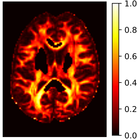
MRtrix3 FA
