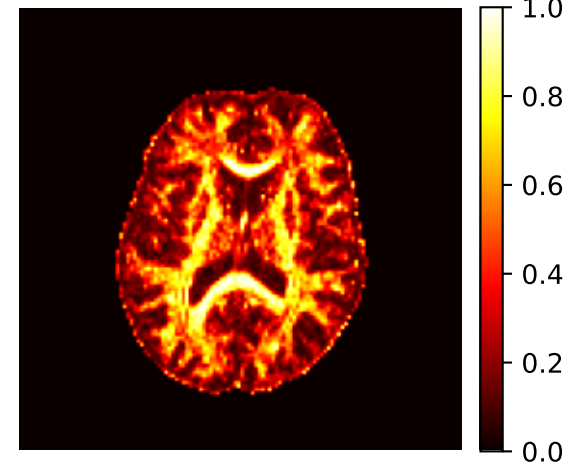
DIPY FA
