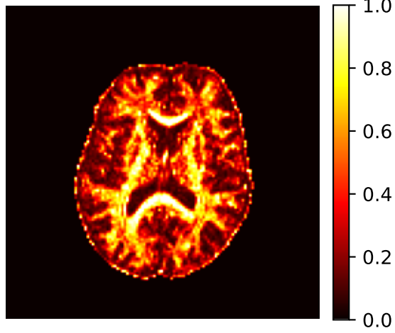
FSL FA
