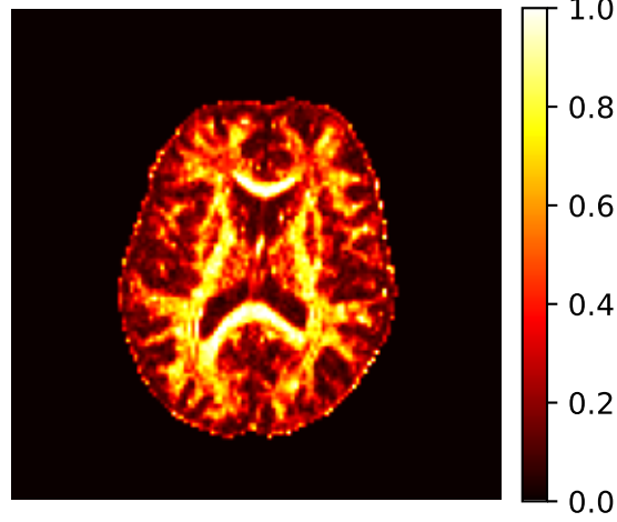
MRtrix3 FA
