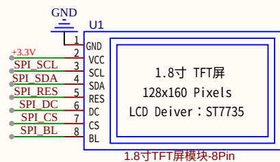
1.8寸TFT屏幕模块
