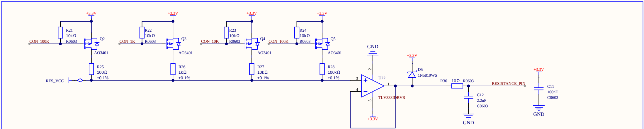
电阻测量电路
