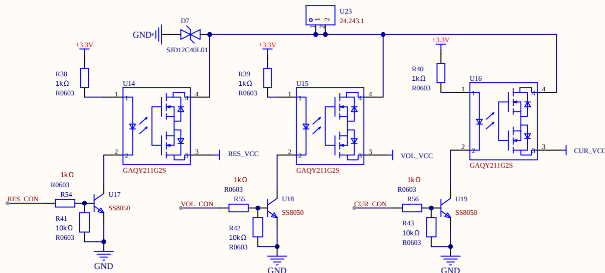
电压电阻选通控制
