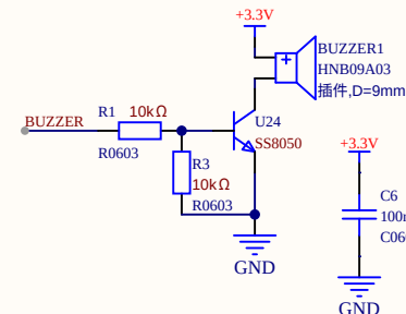
蜂鸣器
