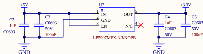
模拟电源
