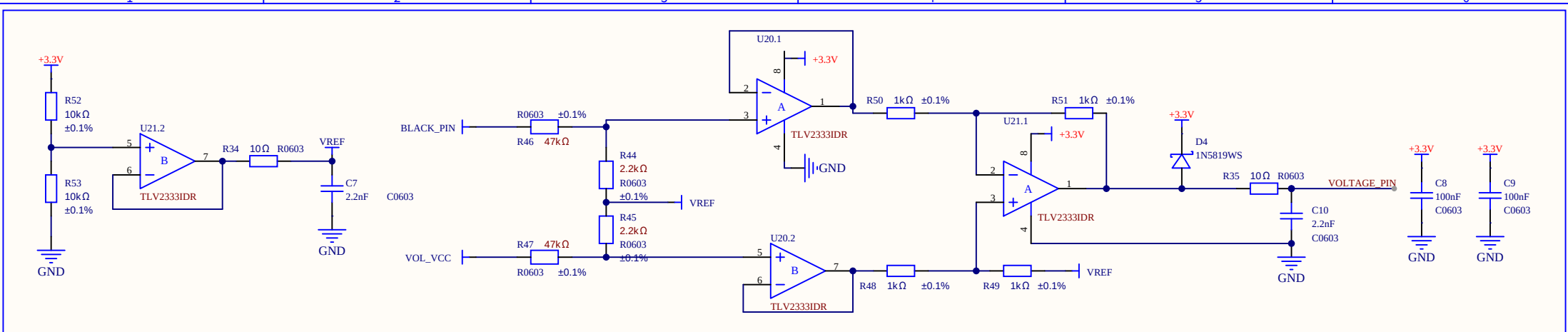
0--36V电压测量电路
