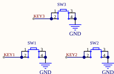
功能按键
