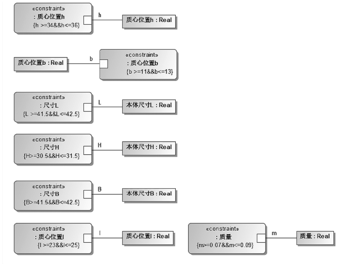
Figure 5-14. Star-sensor parameters
