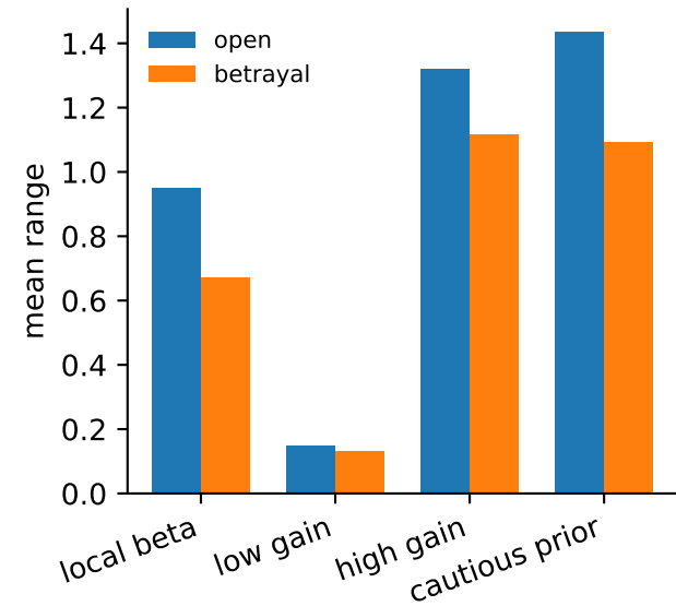
Beta range
