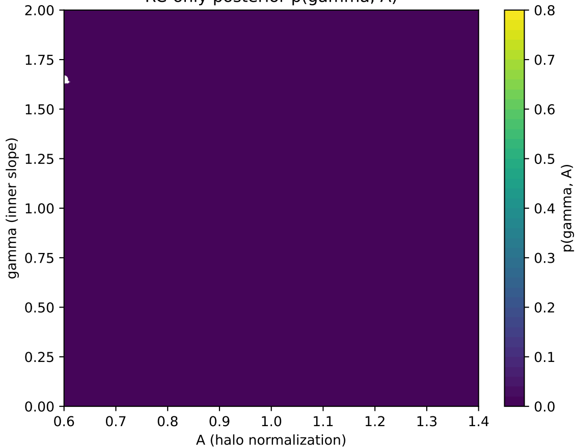
RC-only posterior p(\text{gamma}, A)
