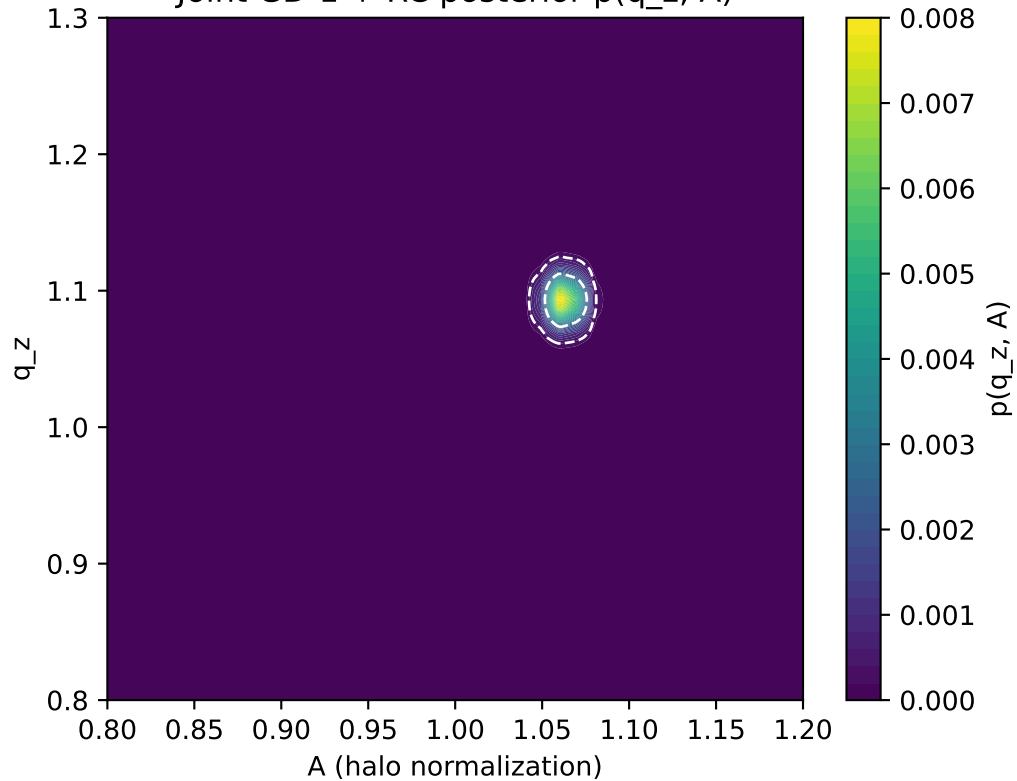
Joint GD-1 + RC posterior p(q_z, A)
