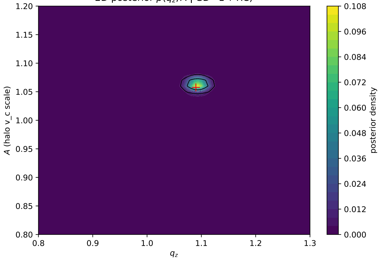
2D posterior p(q_z, A \mid \text{GD-1 + RC})
