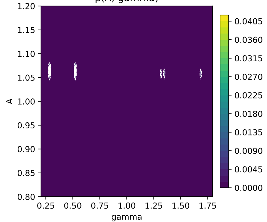
p(A, \text{gamma})
