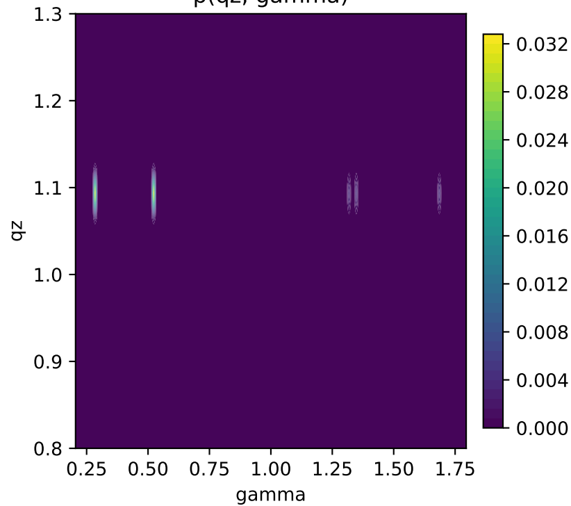
p(qz, \text{gamma})
