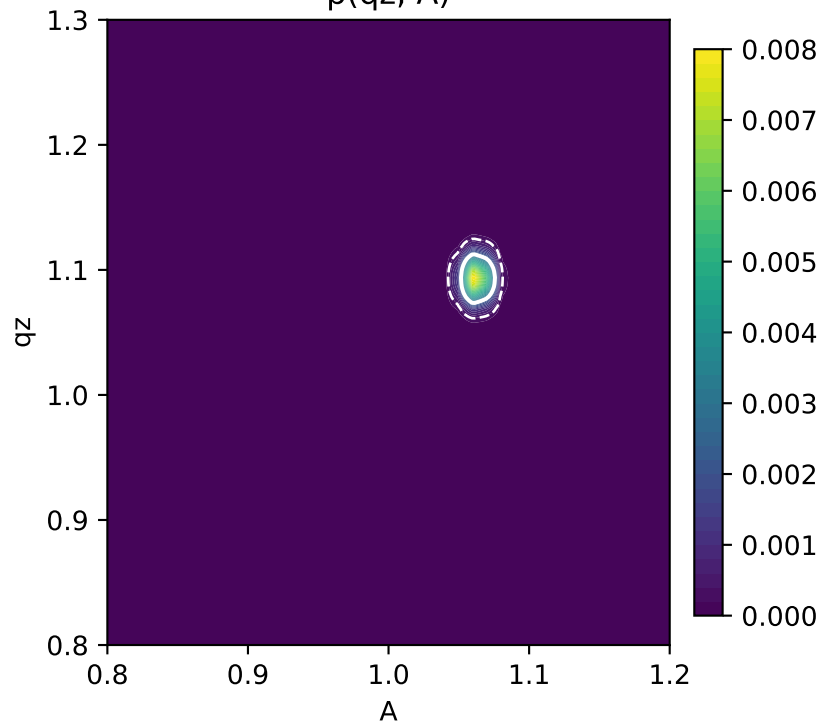
p(qz, A)
