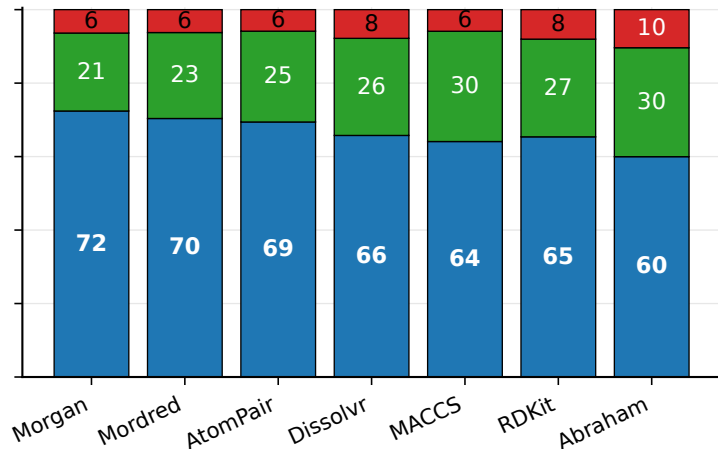
ood split
