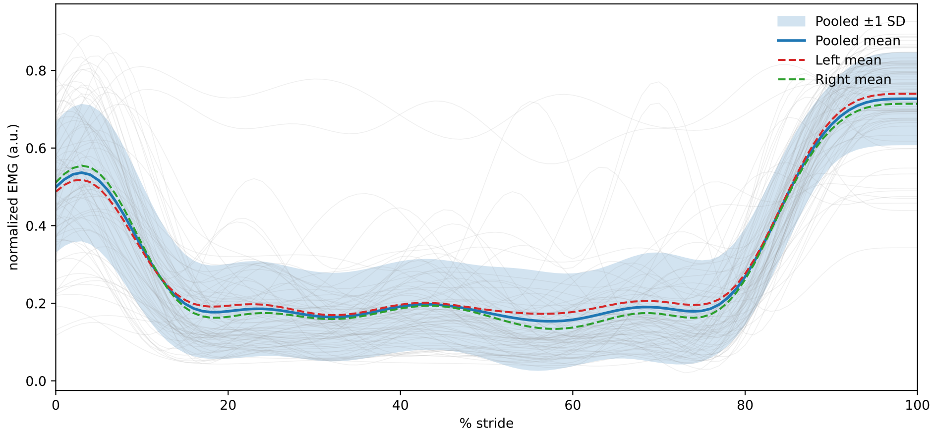
biceps_femoris (n_traces=78)
