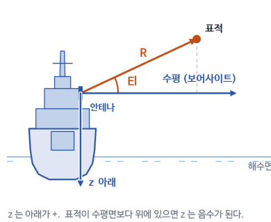
(b) 뒤에서 본 그림 — 고각 티 (Elevation) 같은 배를 선미 쪽에서 본 모습. 수평면에서 위로 잰 각
