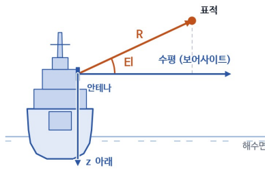
(b) 뒤에서 본 그림 — 고각 티 (Elevation) 같은 배를 선미 쪽에서 본 모습. 수평면에서 위로 잰 각
