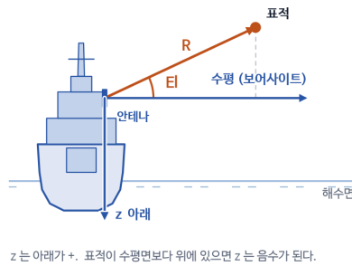
(b) 뒤에서 본 그림 — 고각 E (Elevation) 같은 배를 선미 쪽에서 본 모습. 수평면에서 위로 잰 각
